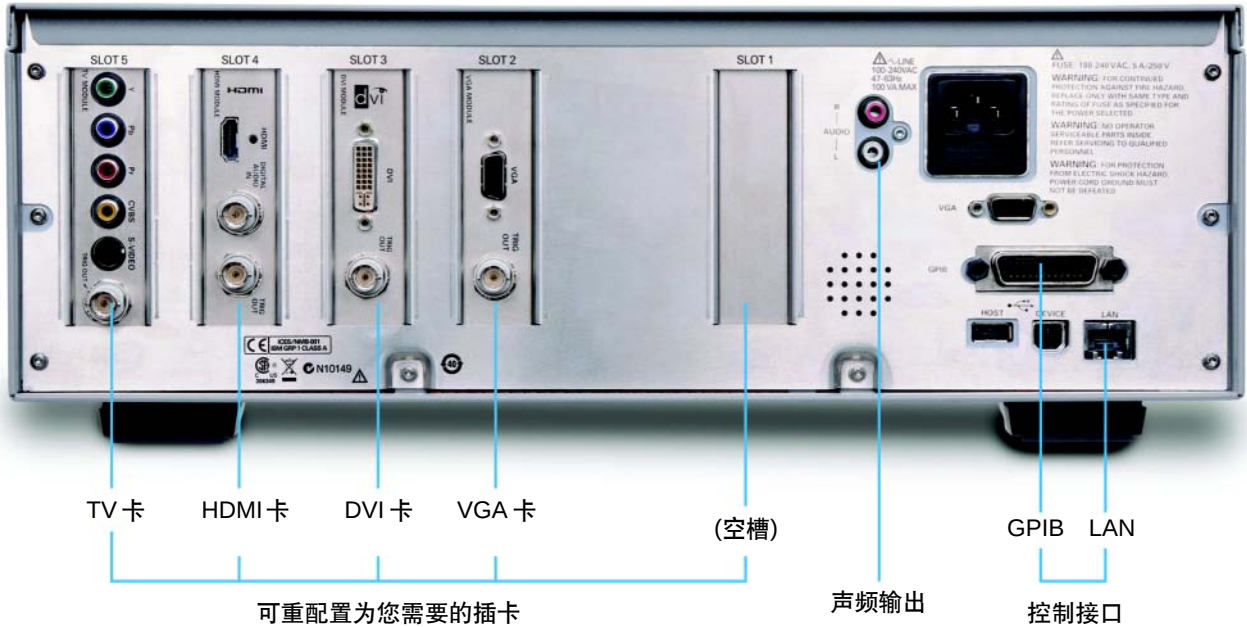
图 7. U8101A 后面板
