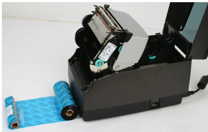
图 2-25. 完全抬起的打印头机构
