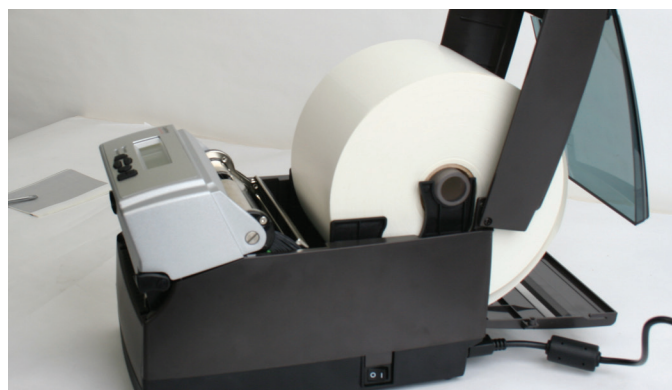
图 2-60. 大介质卷筒安放就位
