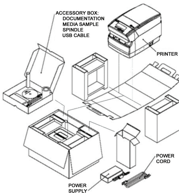
图 2-11. 包装图
