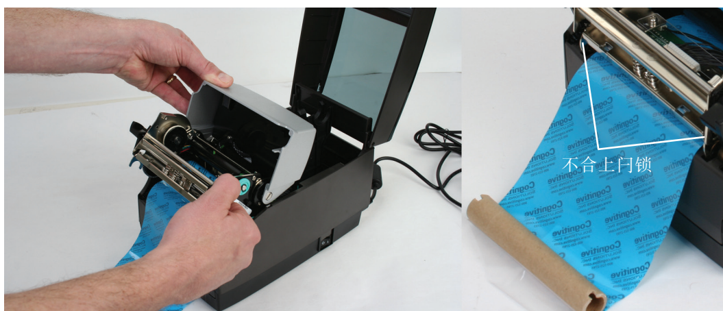
图 2-31. 在不闭上打印头机构的情况下将该机构与用户界面分离，并向下放。
