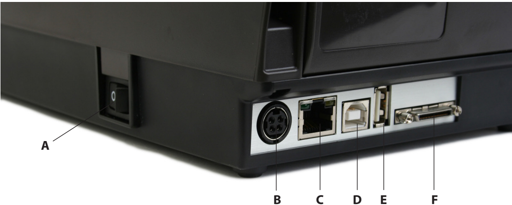
图 2-13. ( 后视图 ) 连接和电源
