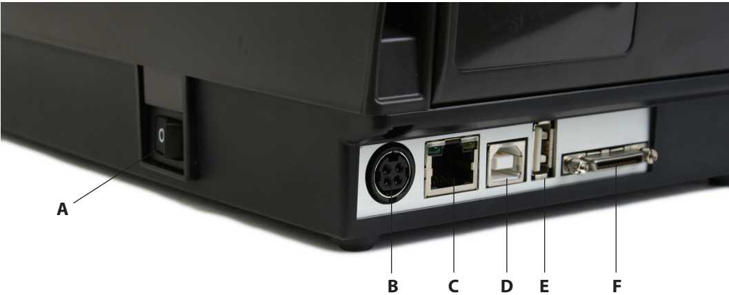
图 5-1. C 系列连接包括 USB A 主机端口
