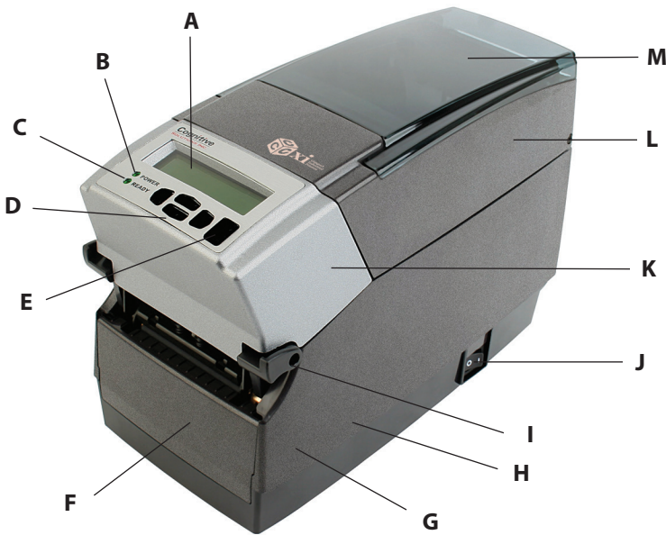
图 2-1. C 系列顶视图和前视图
