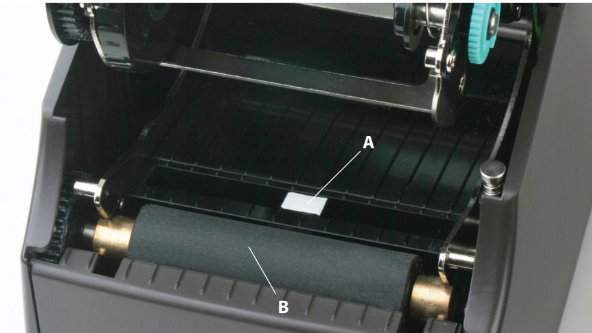
图 2-9. 滚筒总成和标引传感器
