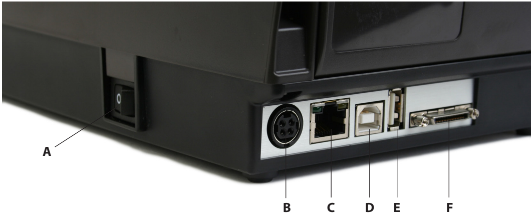
图 2-5. C 系列连接和电源（后视图）
