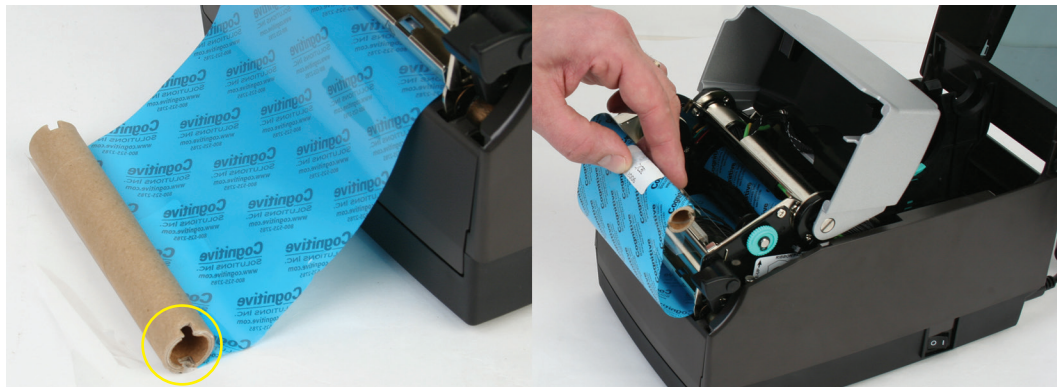
图 2-32. 卷取卷筒槽口和装载卷取卷筒
