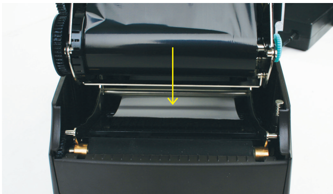
图 2-48. 装载到介质导向装置下的介质的前视图
