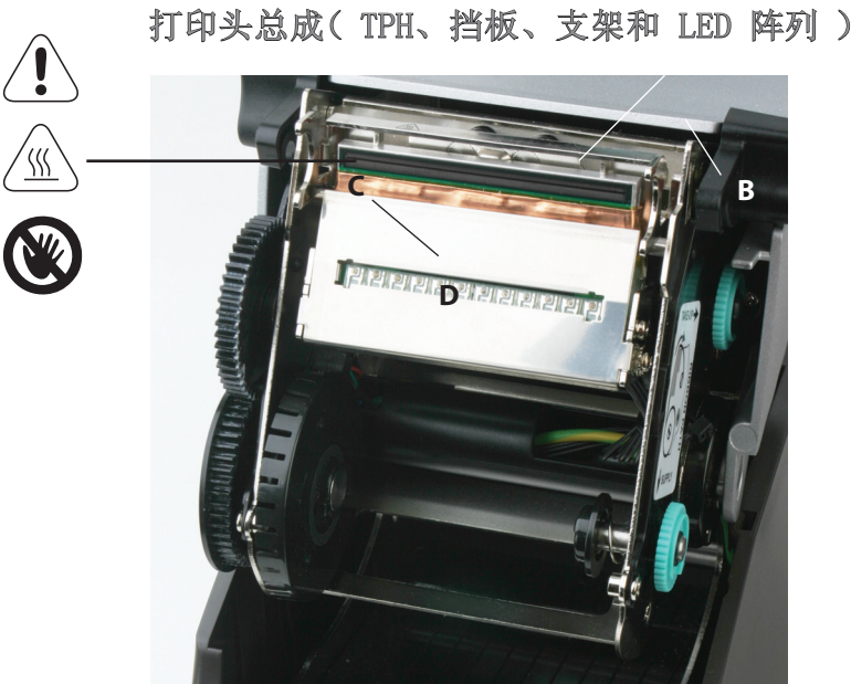
图 2-8. 打印头总成
