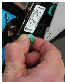
图 2-28. 向外拉色带卷轴
