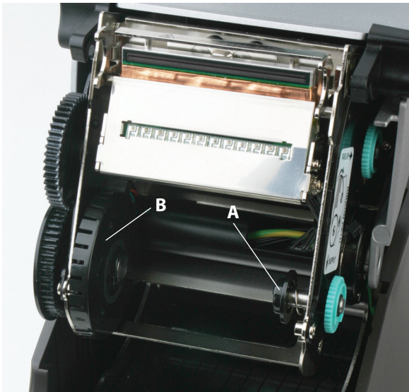
图 2-7. 卷轴和离合器
