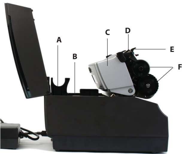
图 2-2. C 系列侧视图
