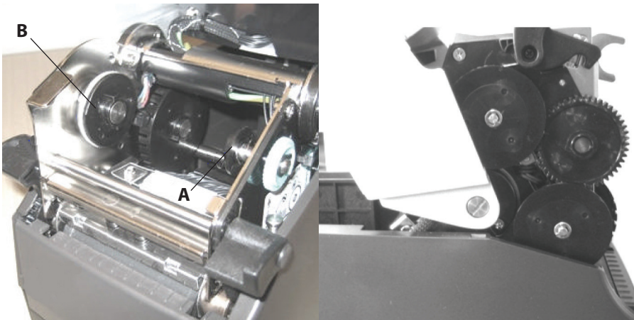
图 2-6. 卷轴、离合器和离合器齿轮侧视图
