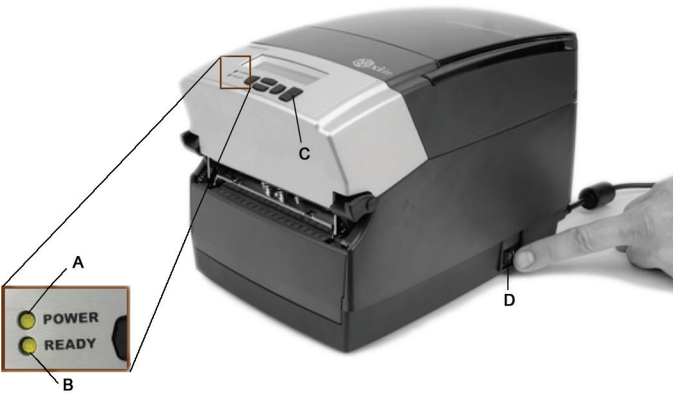
图 2-17：将 C 系列打印机通电
