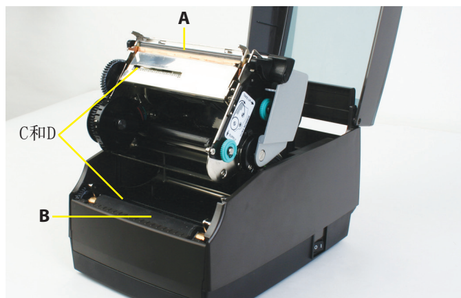
图 12-2. 清洁 C 系列打印机零件
