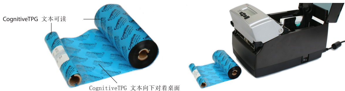
图 2-23. 色带装载到打印机之前色带的放置图
