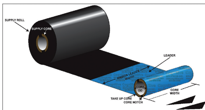
图 10-1. 色带规格图
