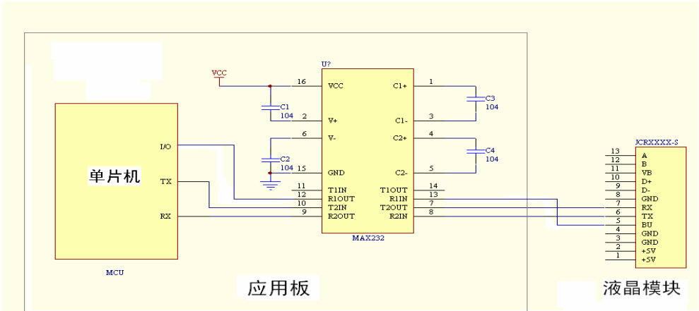
RS232接口参考设计 (带忙线)
