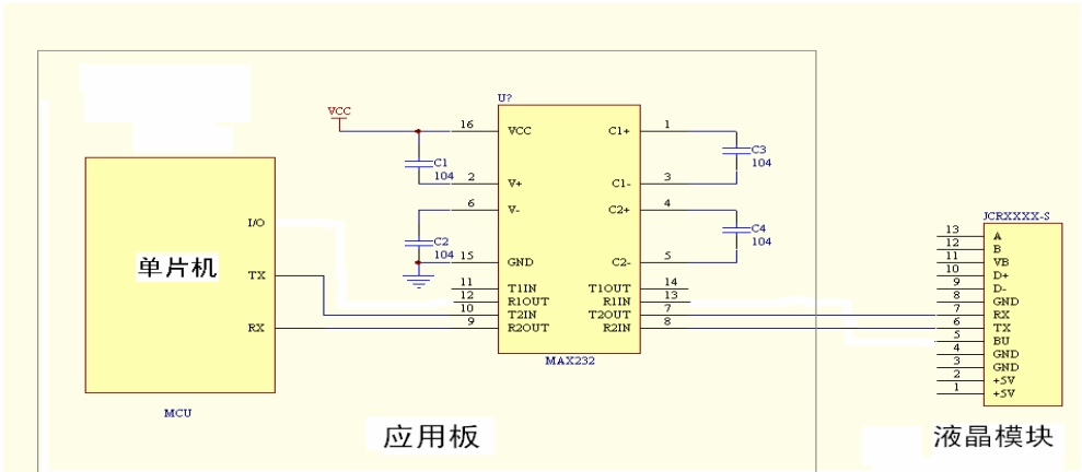
RS232接口参考设计
