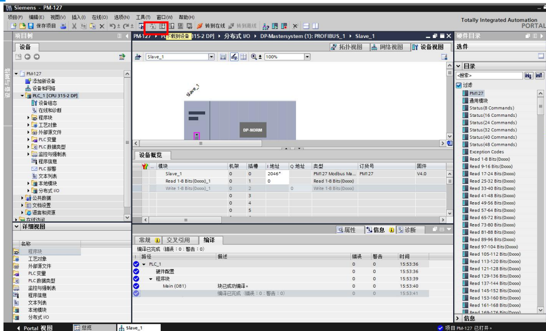
图 24 编译下载
