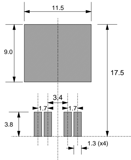
Fig.39. SOT426
