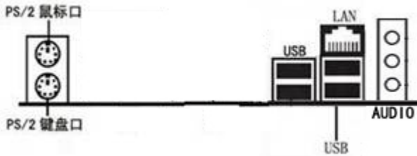
网驰 A770 TWIN V14B 主板 IO 图
