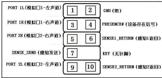
HD Audio 前置音频连接引脚定义
