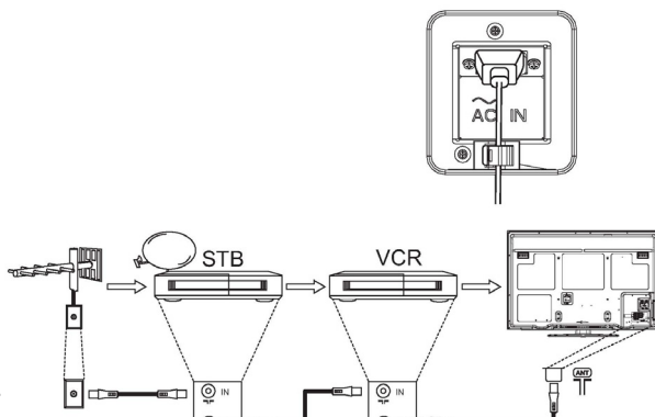
【示例：通过 STB 和 VCR 连接天线】
