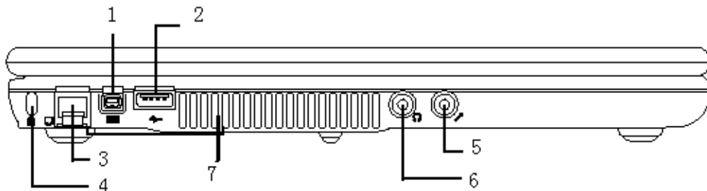
左视图
