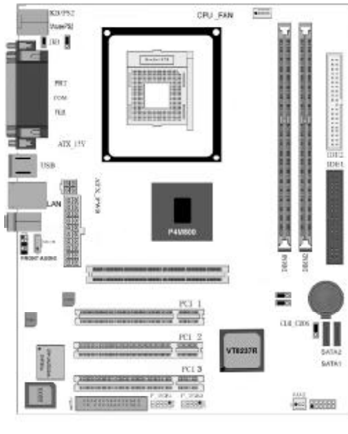
主机板布局图
