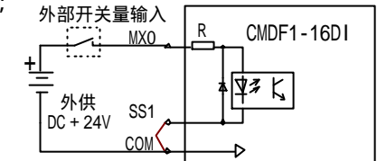
图 4b 源输入电原理框图
