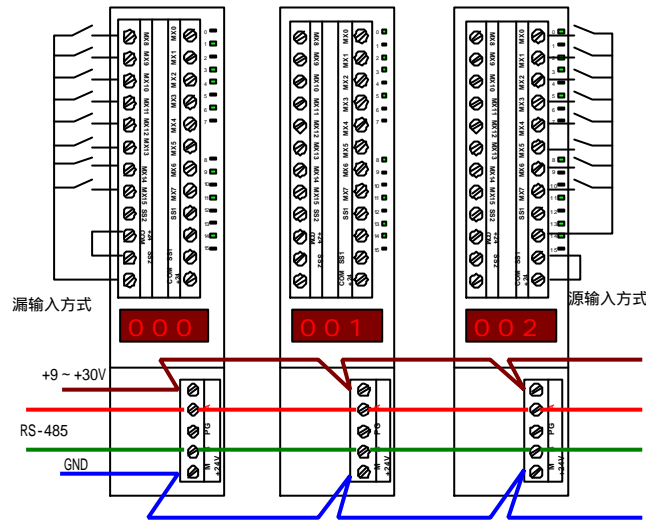
(图 7) CMDF1-16DI 接线参考示意图
