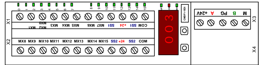
(图 5) CMDF1-16DI 端子示意图
