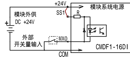
图 4a 漏输入电原理框图
