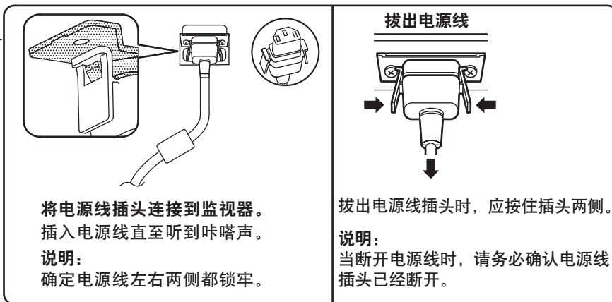
电源线固定方式
