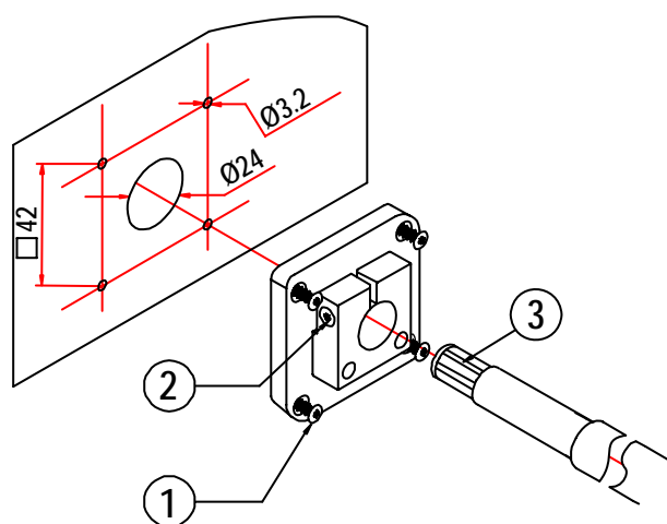
図8 孔あけ指示事項
