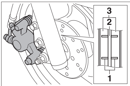
1. 磨耗指示器
