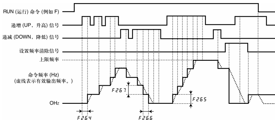
<<采样时序图 2：以脉冲信号进行调整>>
