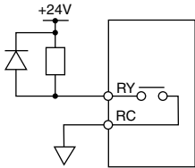
继电器输出端子连接举例
