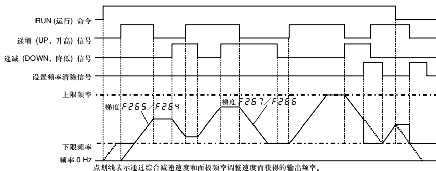
<<采样时序图 1：以连续信号进行调整>>
