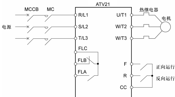
初级回路内接触器的连接举例
