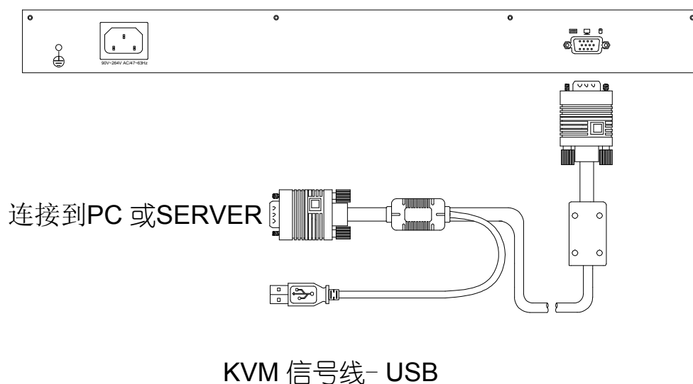
图 2-3（信号线及其连接）
