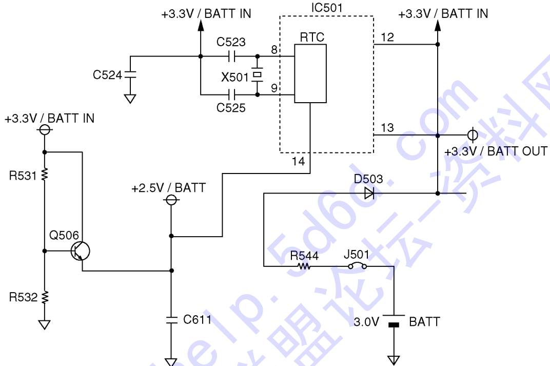
电路图
