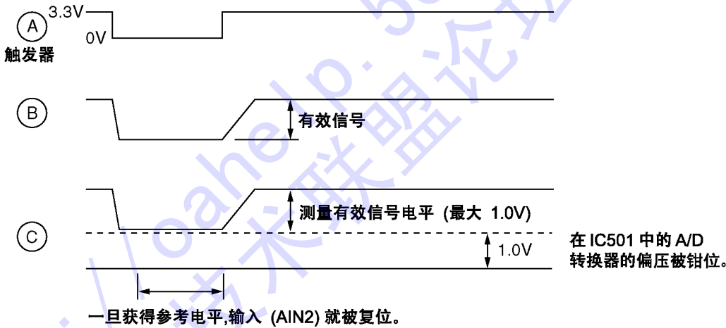
计时图
