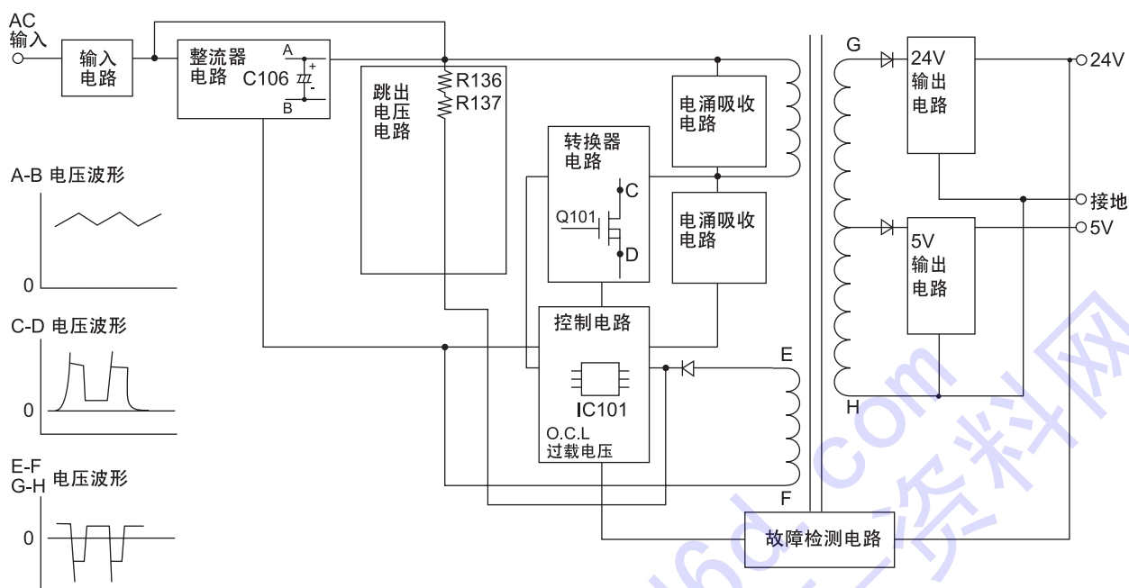
方框图
