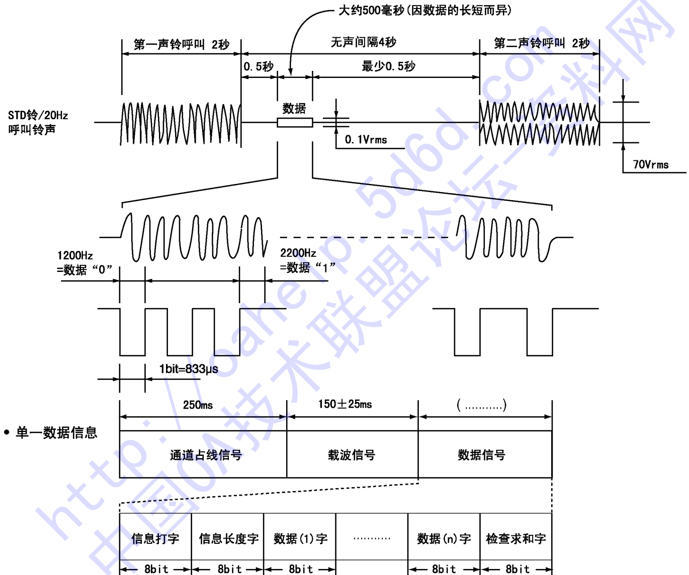
定时图
