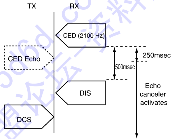
图 b (通过改变 CED 频率的对策)
