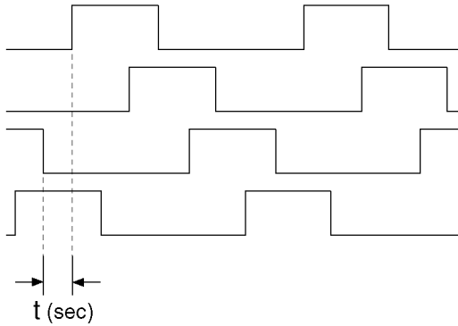
步进马达定时图
