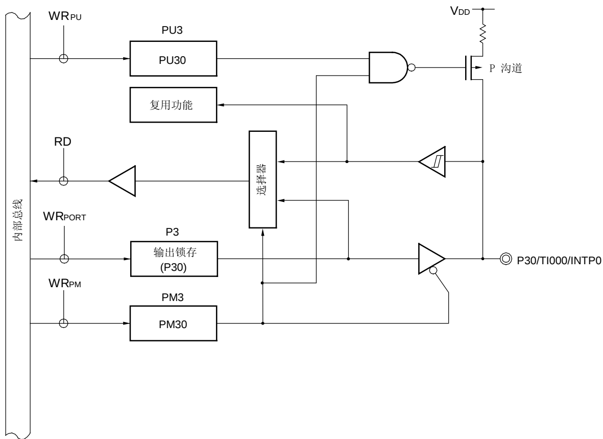
图 4-4 P30 的框图
