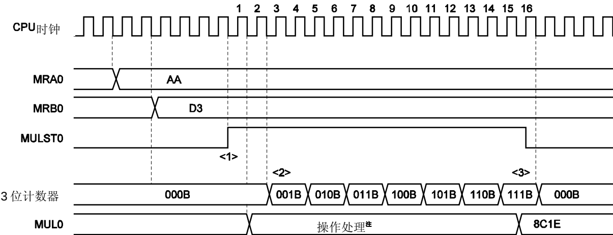
图 12-3. 乘法器操作时序 (示例为 AAH × D3H)
