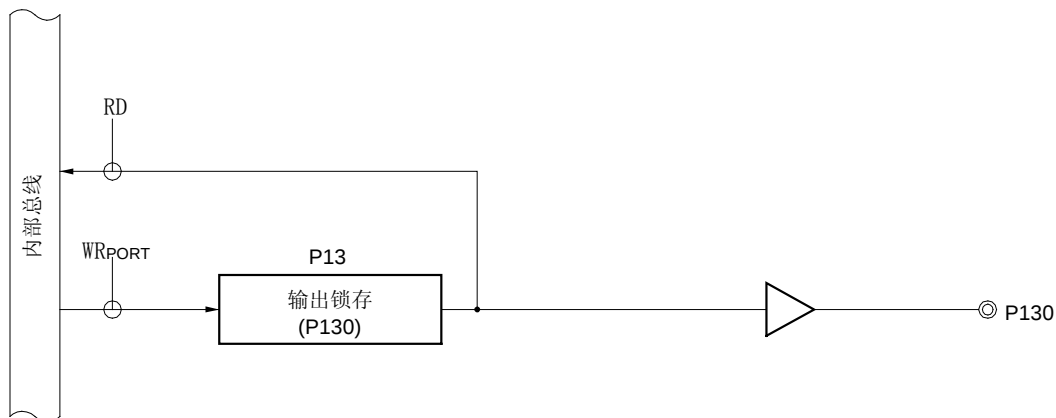
图 4-14. P130 的框图
