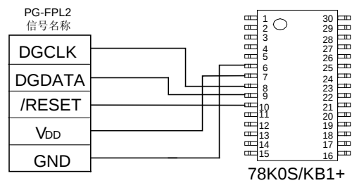
图 19-5. 与 PG-FPL2 的连线图
