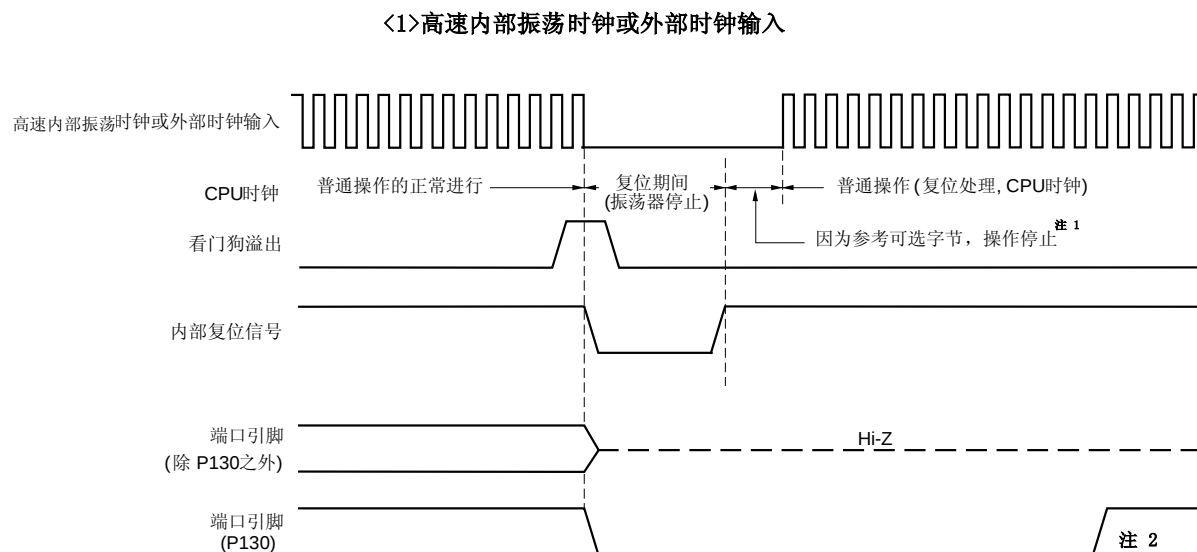
图 15-3. 由看门狗定时器溢出引起的复位时序
