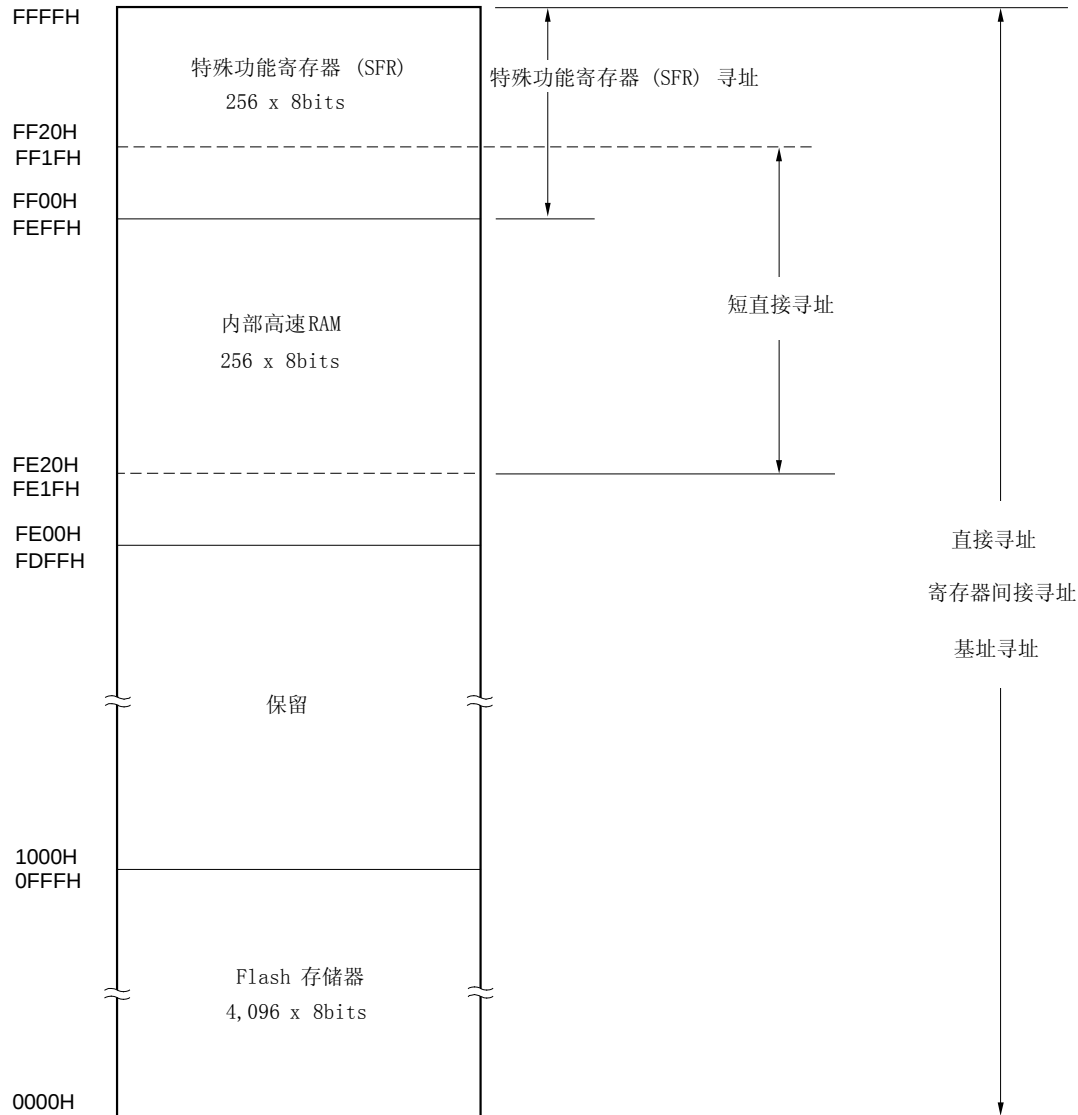
图 3-3. 数据存储器寻址(μPD78F9232)
