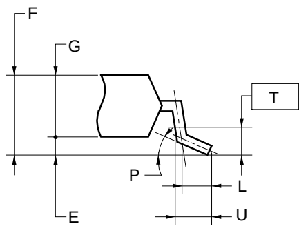
引脚端详图
