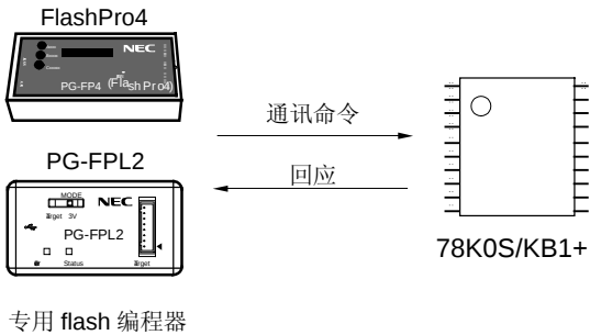
图 19-9. 通讯命令
