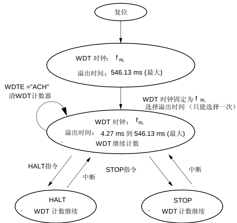
图 9-4. 当由选项字节选择“低速内部振荡不能被停止”时的状态转换图
