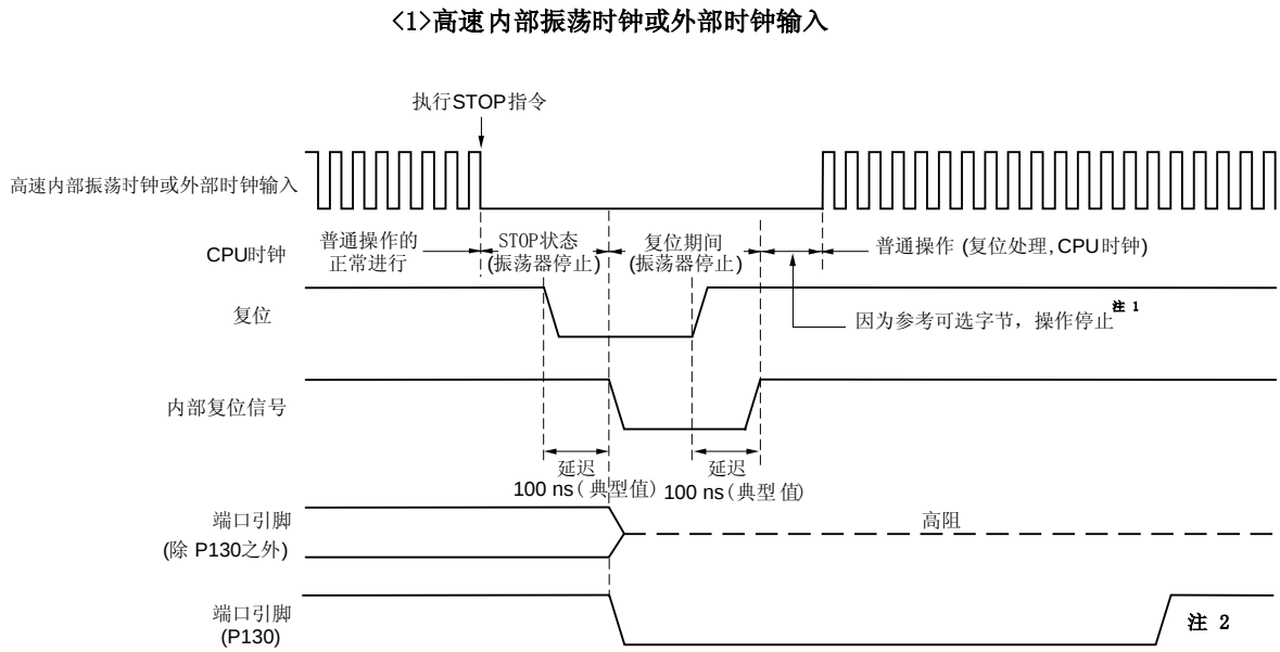
图 15-4. 在 STOP 模式中由 RESET 输入引起的复位时序
