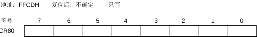
图 7-2. 8 位比较寄存器 80 (CR80) 格式
