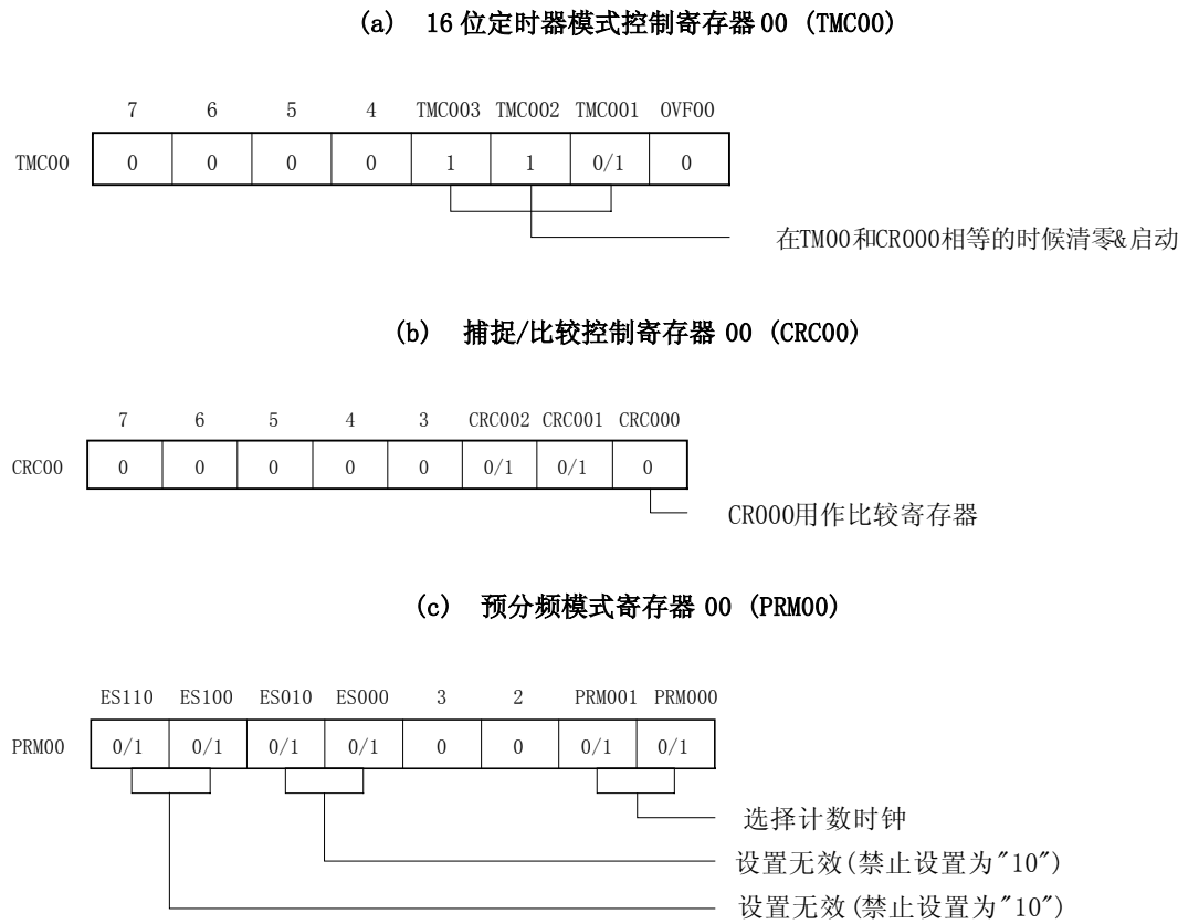
图 6-10. 设置控制寄存器用于时间间隔定时器操作
