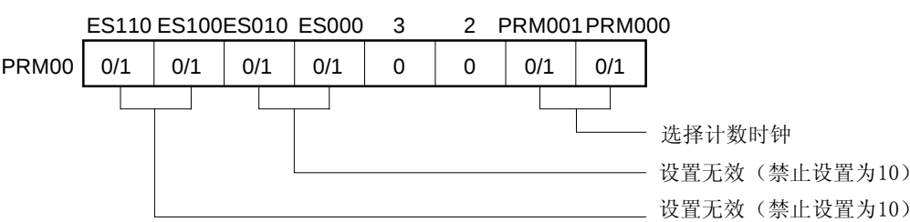
(d) 预分频模式寄存器 00 (PRM00)
