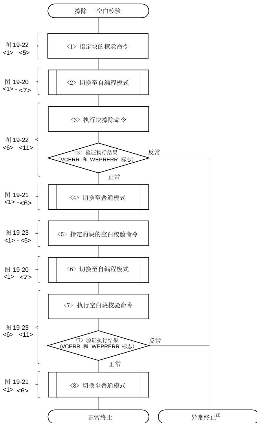
图 19-29. 自编程模式下中断屏蔽时命令执行时间最短的操作流程（从擦除到空白块检验）
