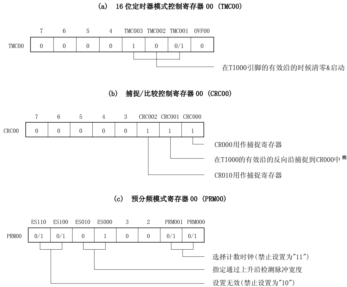
图 6-25. 通过重启定时器设置脉冲宽度测量的控制寄存器（指定上升沿有效）
