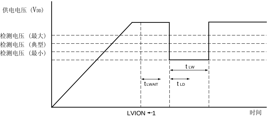
数据存储器 STOP 模式低电源电压下数据保持特性 (TA = -40 ~ +125℃)
