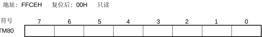
图 7-3. 8 位定时器计数器 80 (TM80) 的格式
