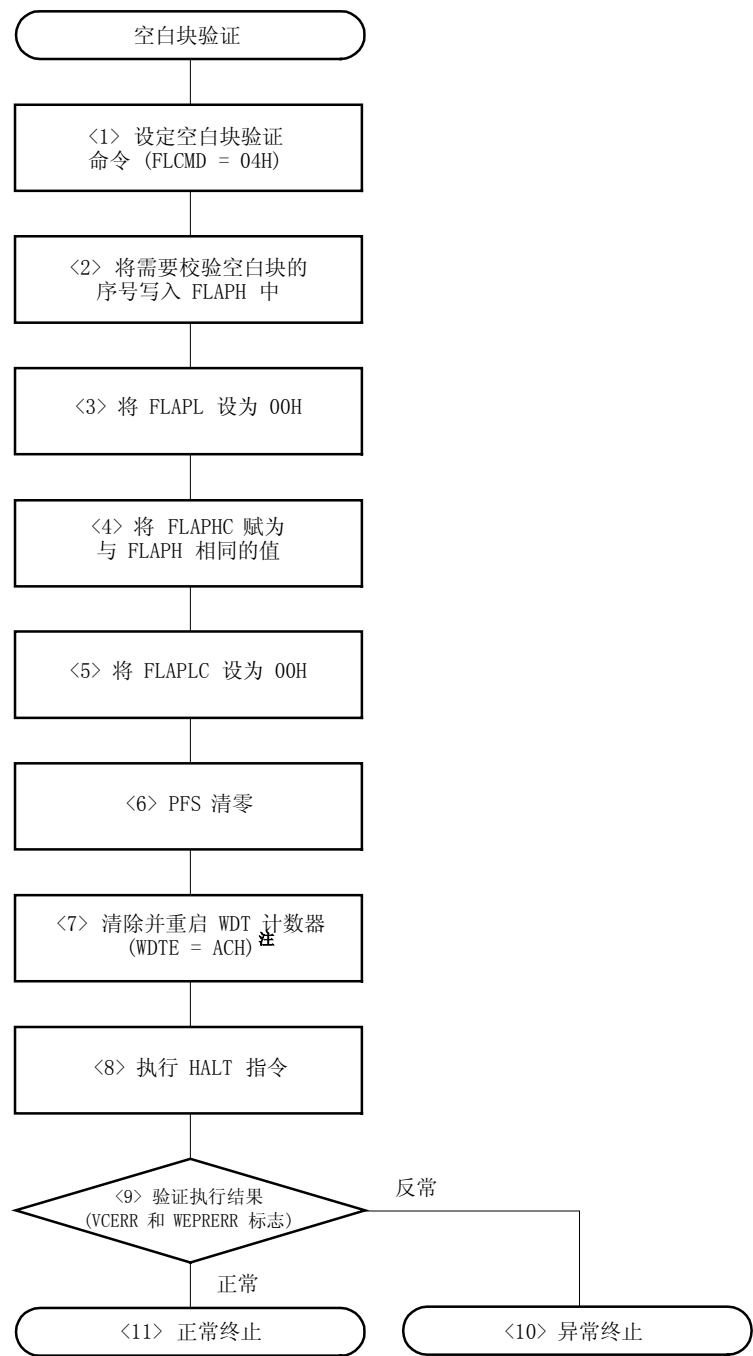
图 19-23. 在自编程模式下 block 空白检测操作流程
