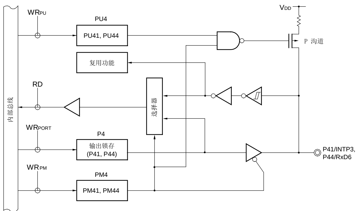
图 4-9. P41 和 P44 的框图
