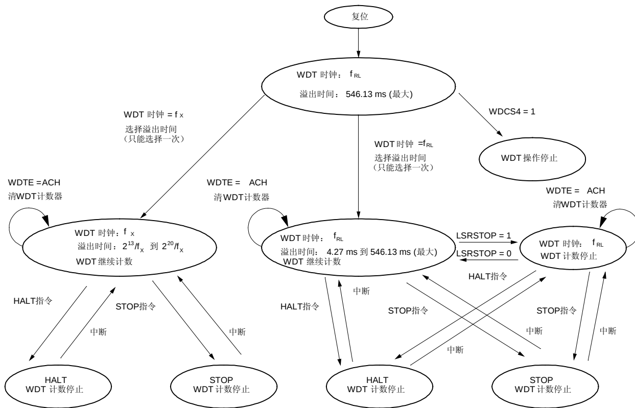
图 9-5. 当由选项字节选择“可通过软件停止低速内部振荡时钟”时的状态转换图
