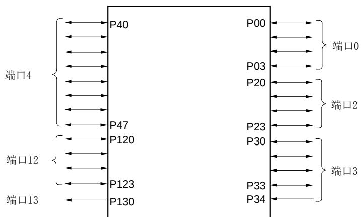
图 4-1. 端口功能
