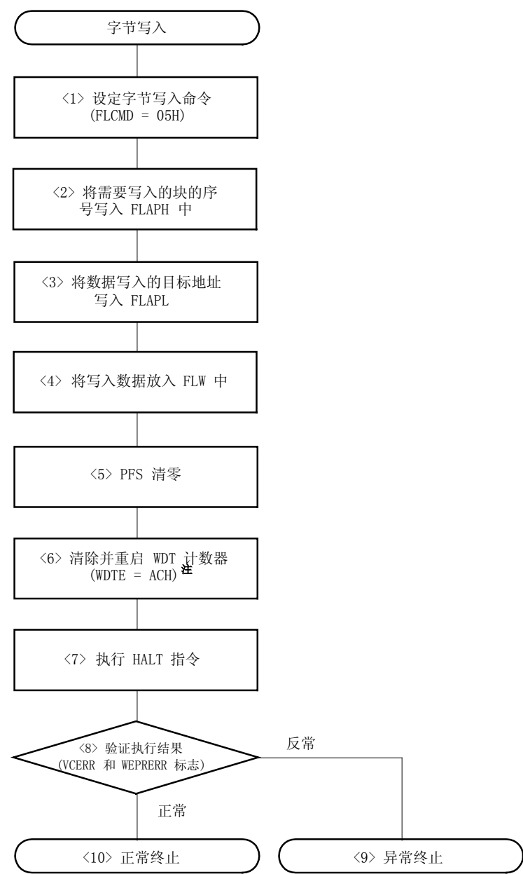
图 19-24. 自编程模式下字节写入操作流程
