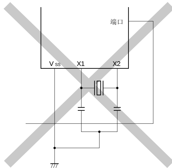
(b) 信号线与振荡器导线互相交叉
