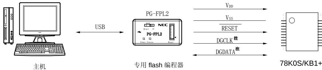
图 19-3. 写入 FLASH 存储器的环境(PG-FPL2)
