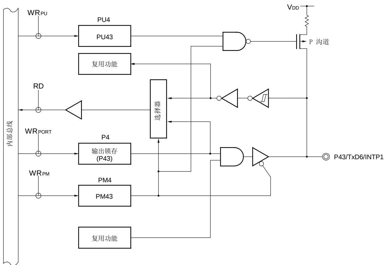
图 4-11. P43 的框图
