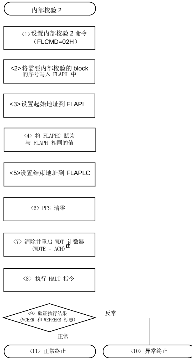
图 19-26. 自编程模式下内部校验 2 流程
