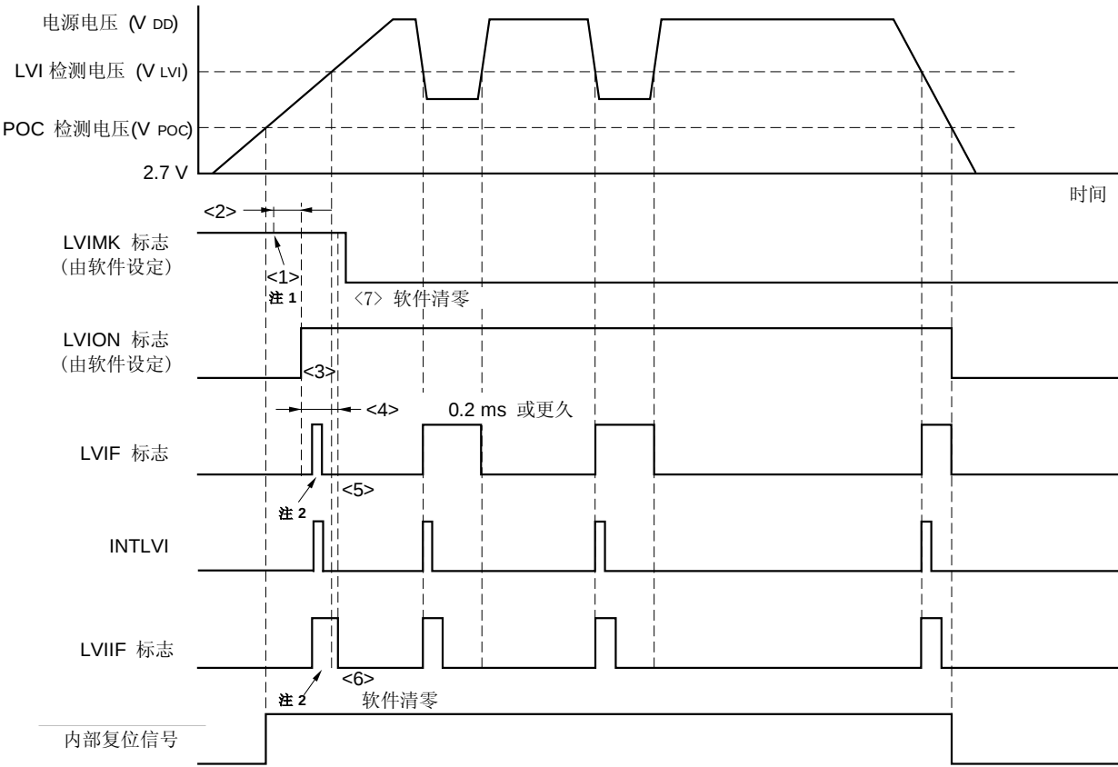
图 17-5. 低电压检测器中断信号产生时序
