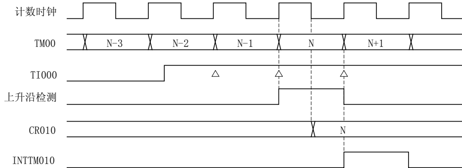
图 6-17. 指定上升沿的 CR010 捕捉操作
