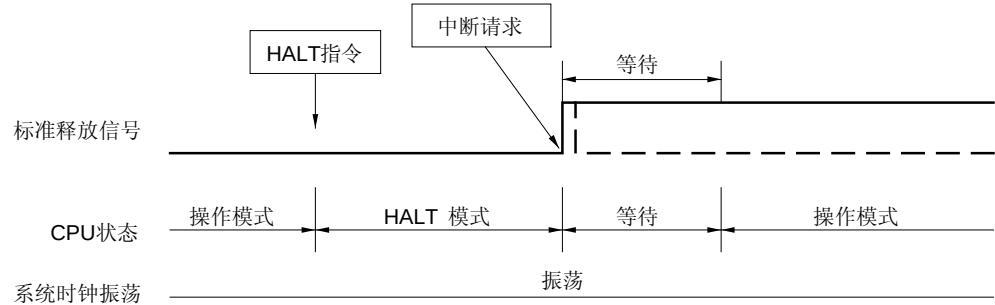
图 14-2. 通过产生中断请求释放 HALT 模式
