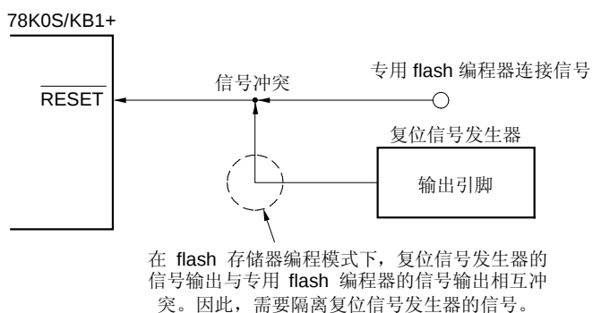
图 19-8. 信号冲突(RESET 引脚)
