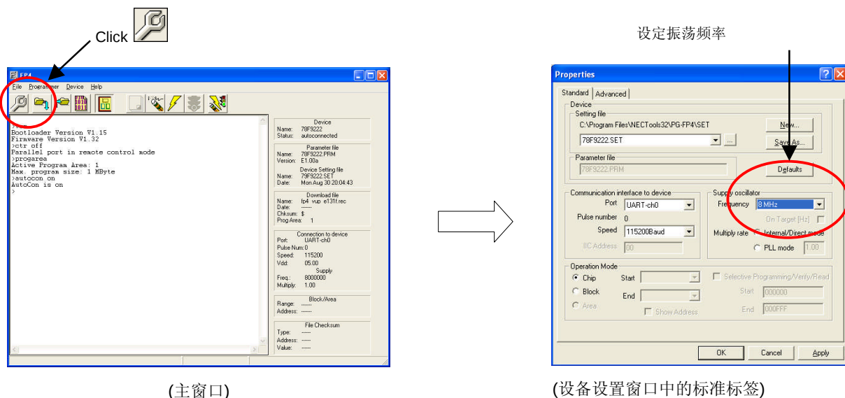
图 19-7. PG-FP4 GUI 软件设置示例
