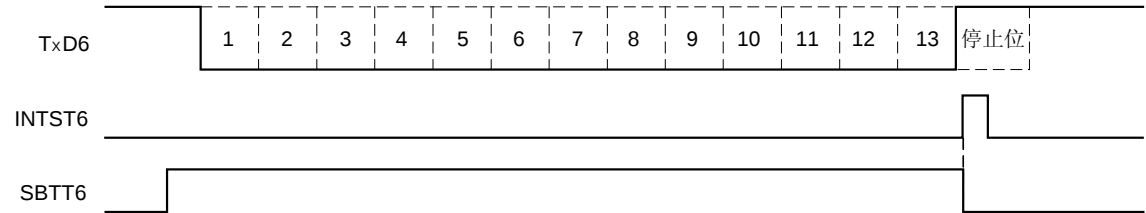
图 11-22. SBF 发送
