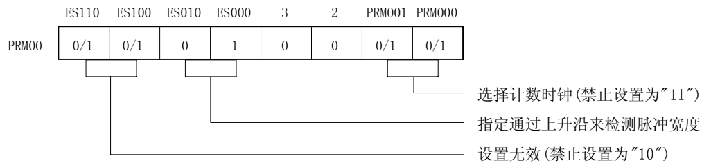
(c) 预分频模式寄存器 00 (PRM00)
