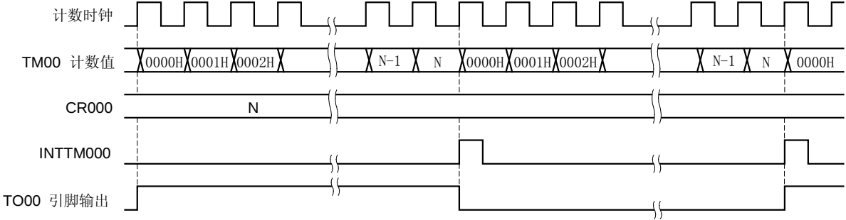
图 6-28. 方波输出操作时序
