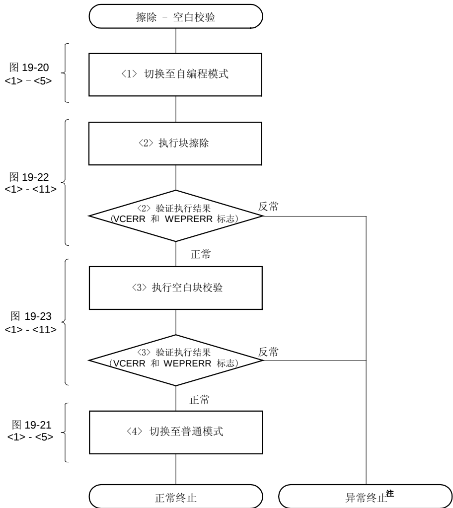
图 19-27 命令执行时间最短的操作流程（从擦除到空白检验）
