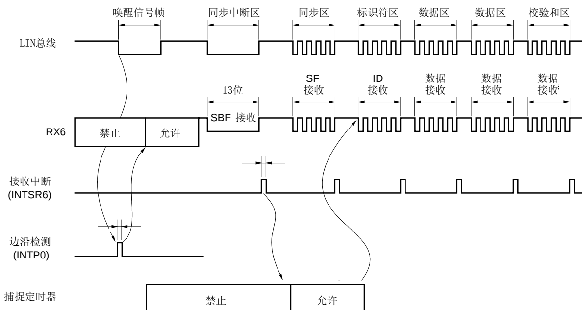
图 11-2. LIN 接收操作
