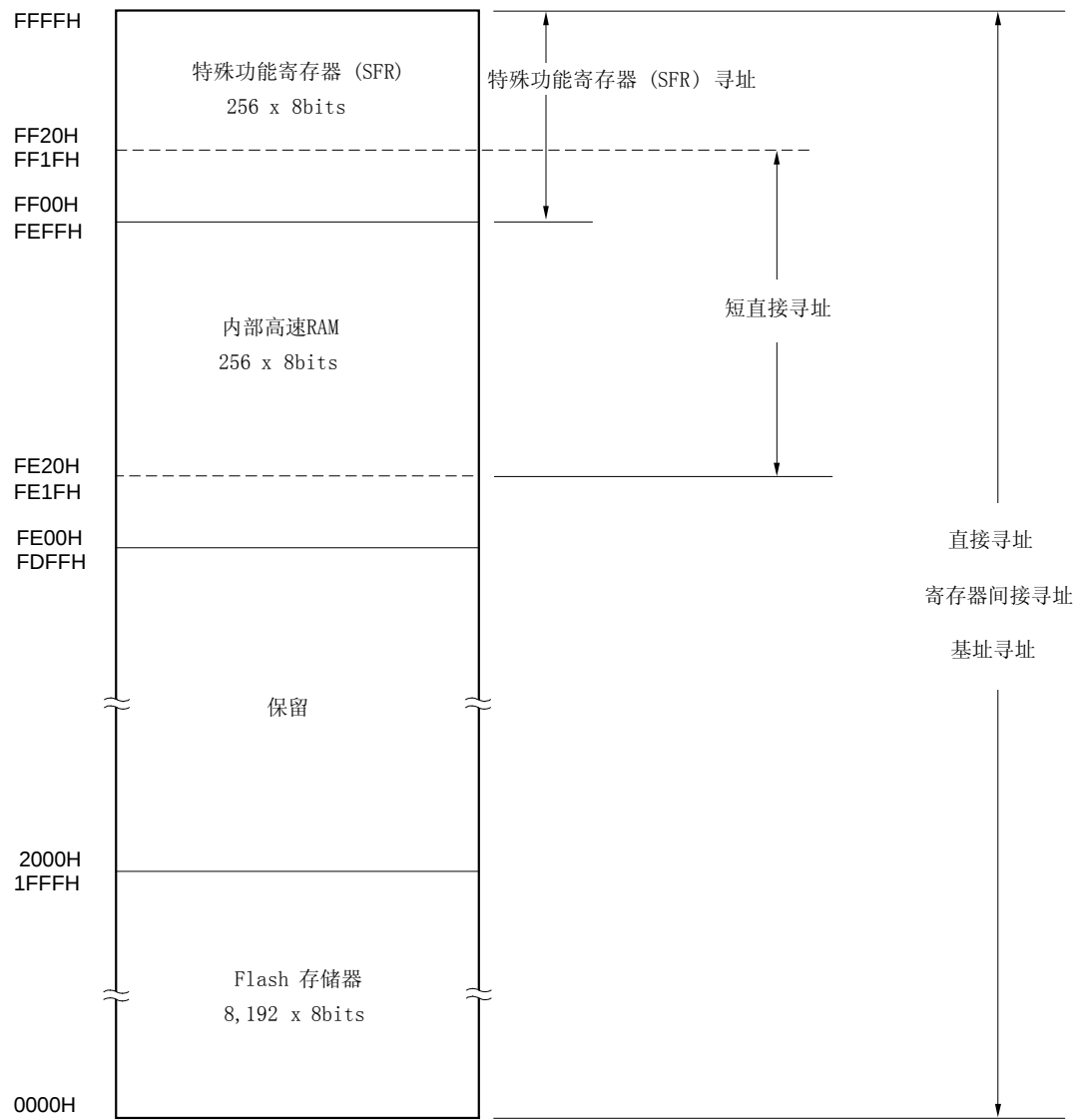
图 3-4. 数据存储寻址( \mu PD78F9234)
