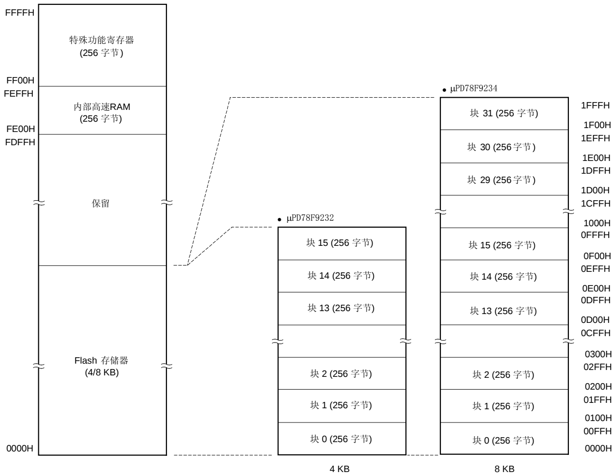
图 19-1. Flash 存储器映射图
