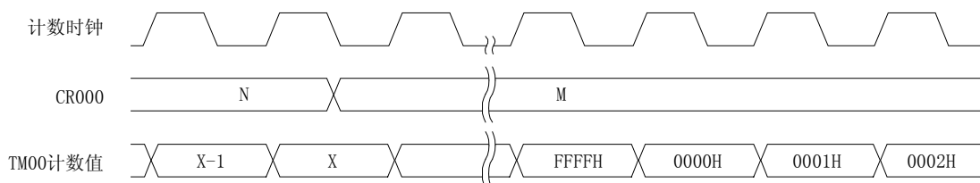
图 6-13. 在定时器计数操作过程中比较寄存器改变之后的时序 ( N \rightarrow M: N > M )
