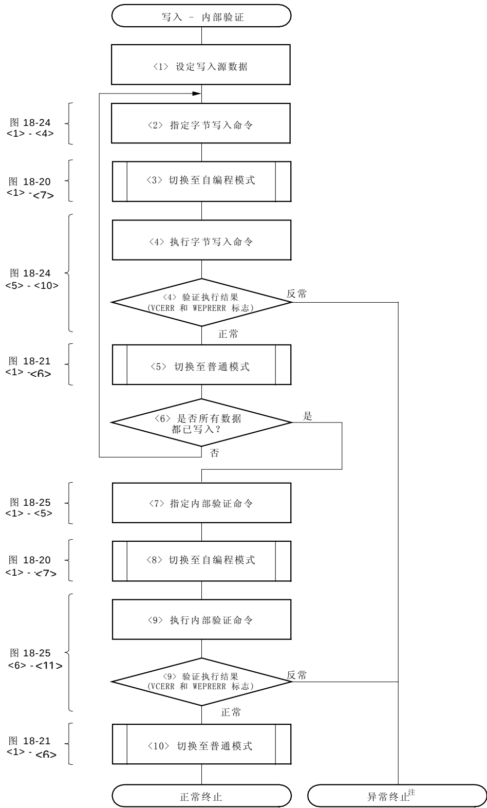
图 19-30. 自编程模式下中断屏蔽时命令执行时间最短的操作流程（从写入到内部校验）
