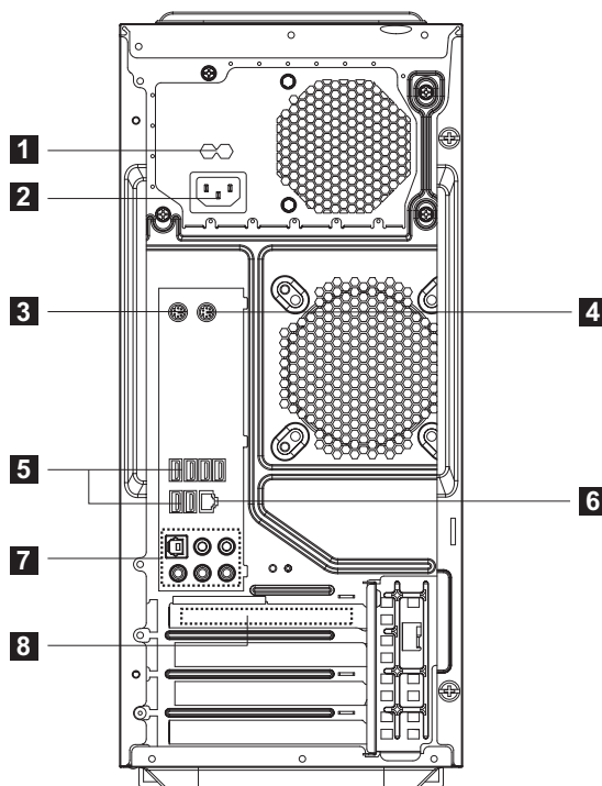
后部接口图 3 (适用于部分机型)
