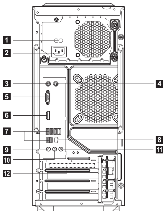
后部接口图 2 ( 适用于部分机型 )
