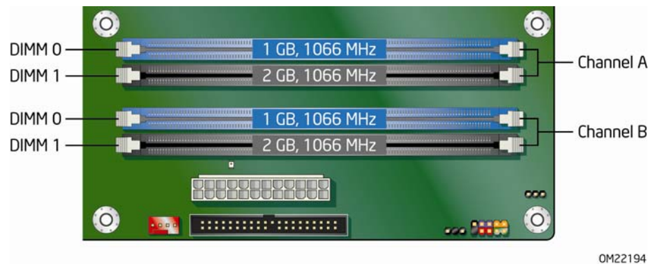
图 14. 四条 DIMM 下双通道内存配置
