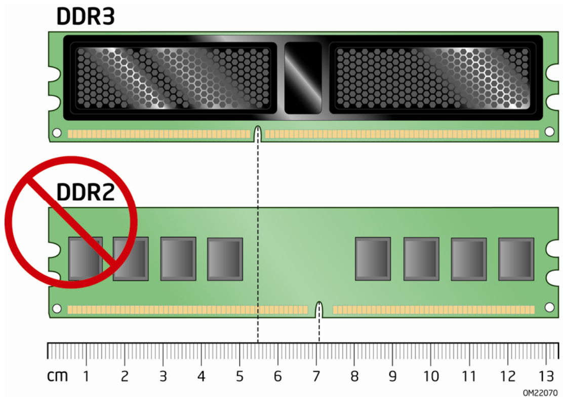
图 16. 使用 DDR3 DIMM
