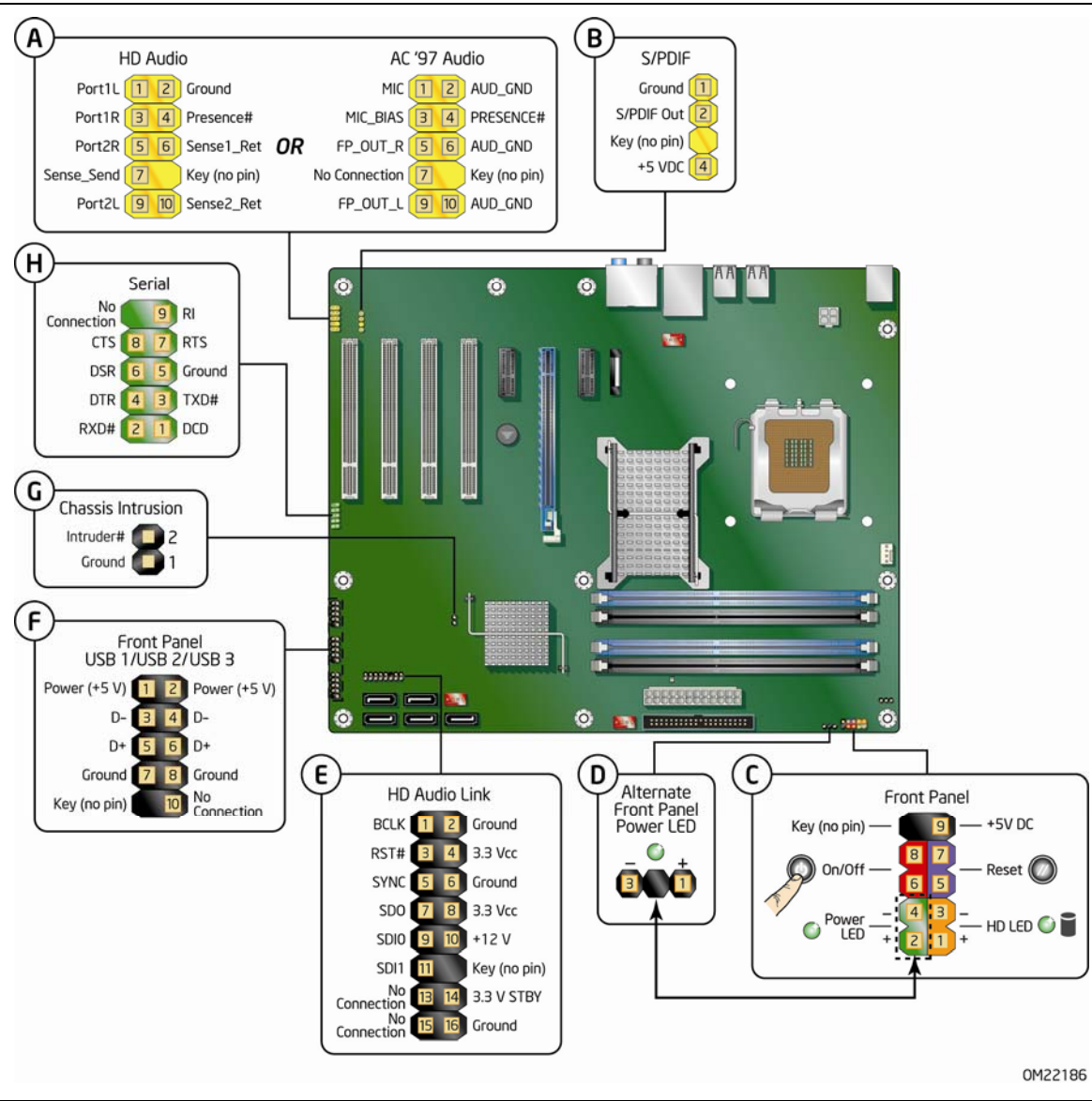
图 22. 内置接头连接器
