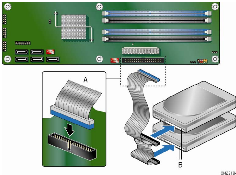
图 20. 连接 IDE 电缆
