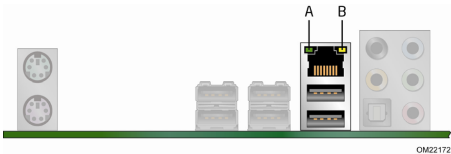
图 2. LAN 状态 LED 指示灯
