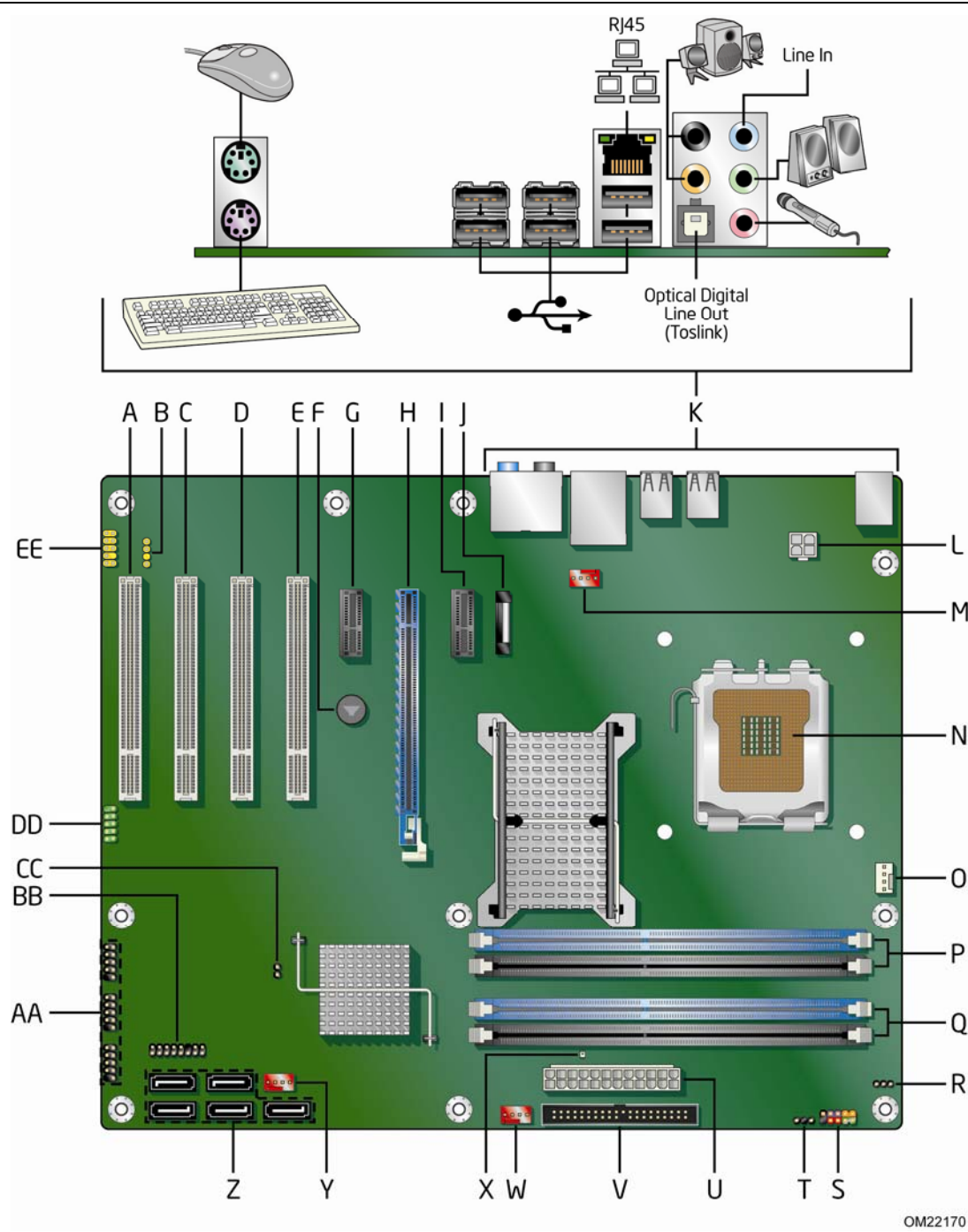
图 1. 英特尔台式机主板 DP43BFL 组件
