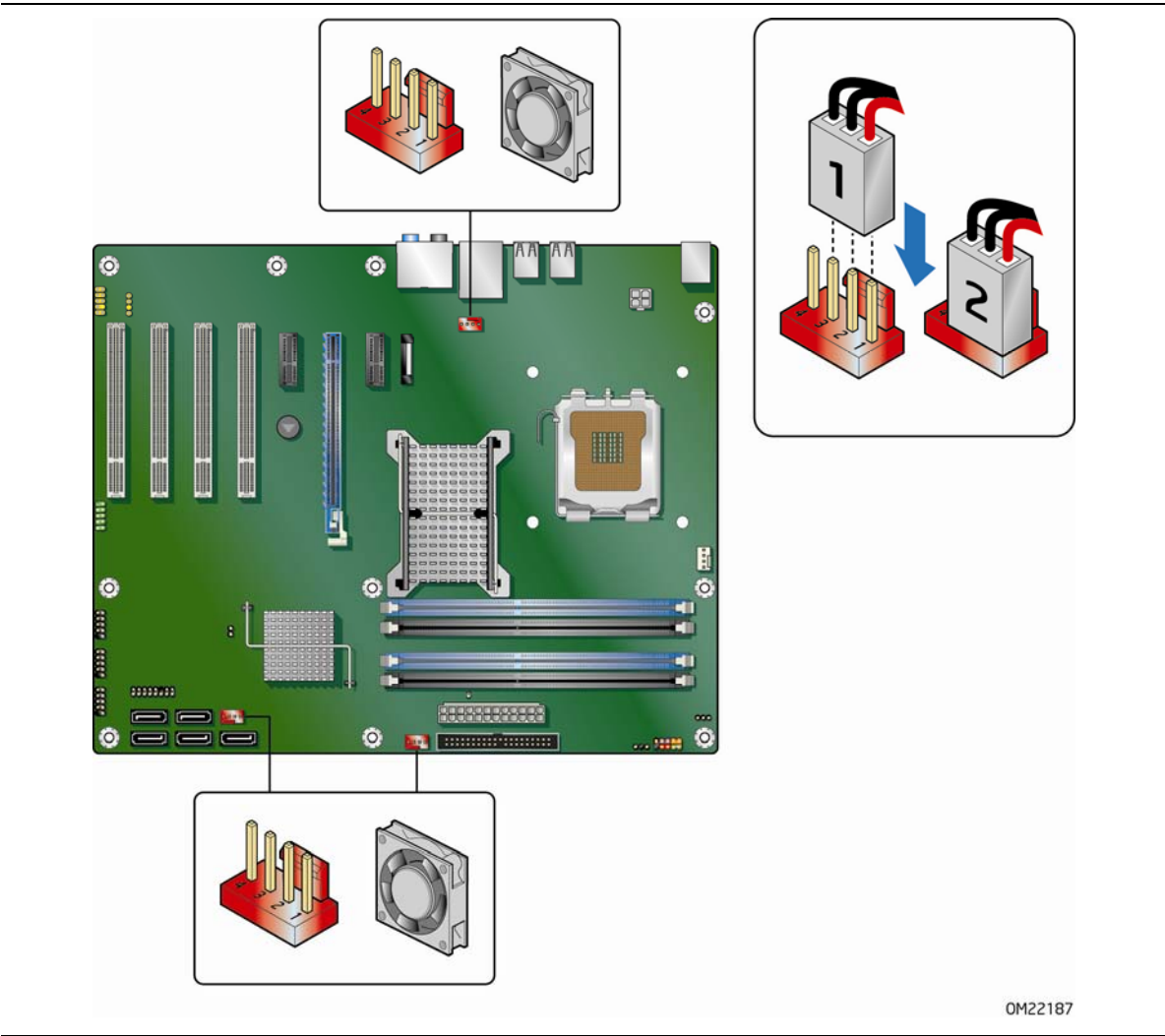
图 24. 机箱风扇接头连接器位置
