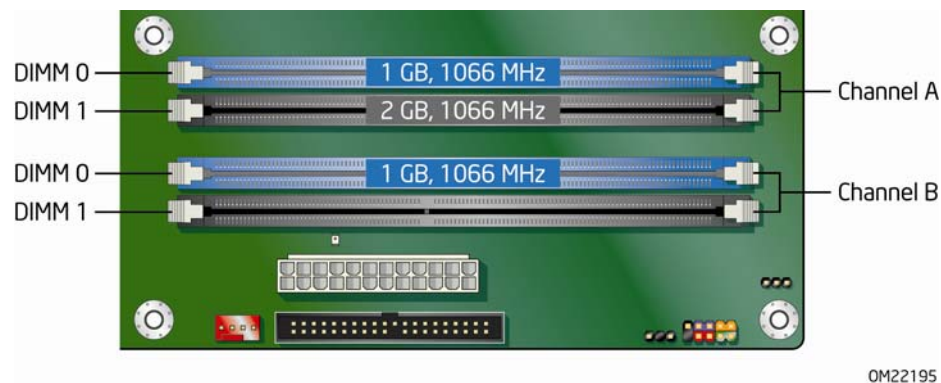
图 15. 三条 DIMM 下双通道内存配置
