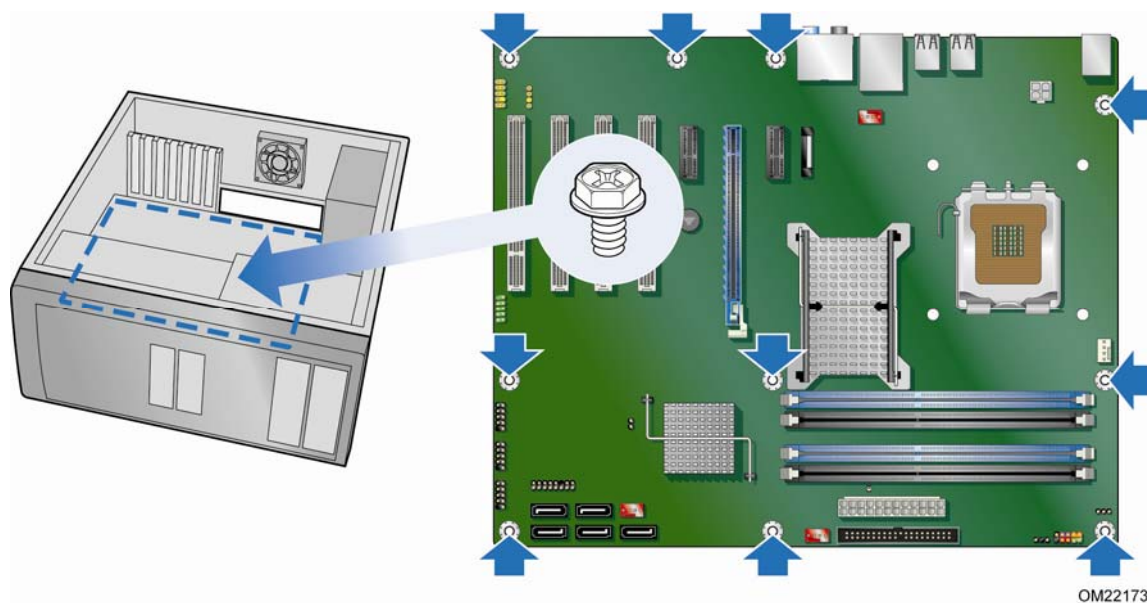
图 5. 英特尔台式机主板 DP43BFL 安装螺丝孔位置
