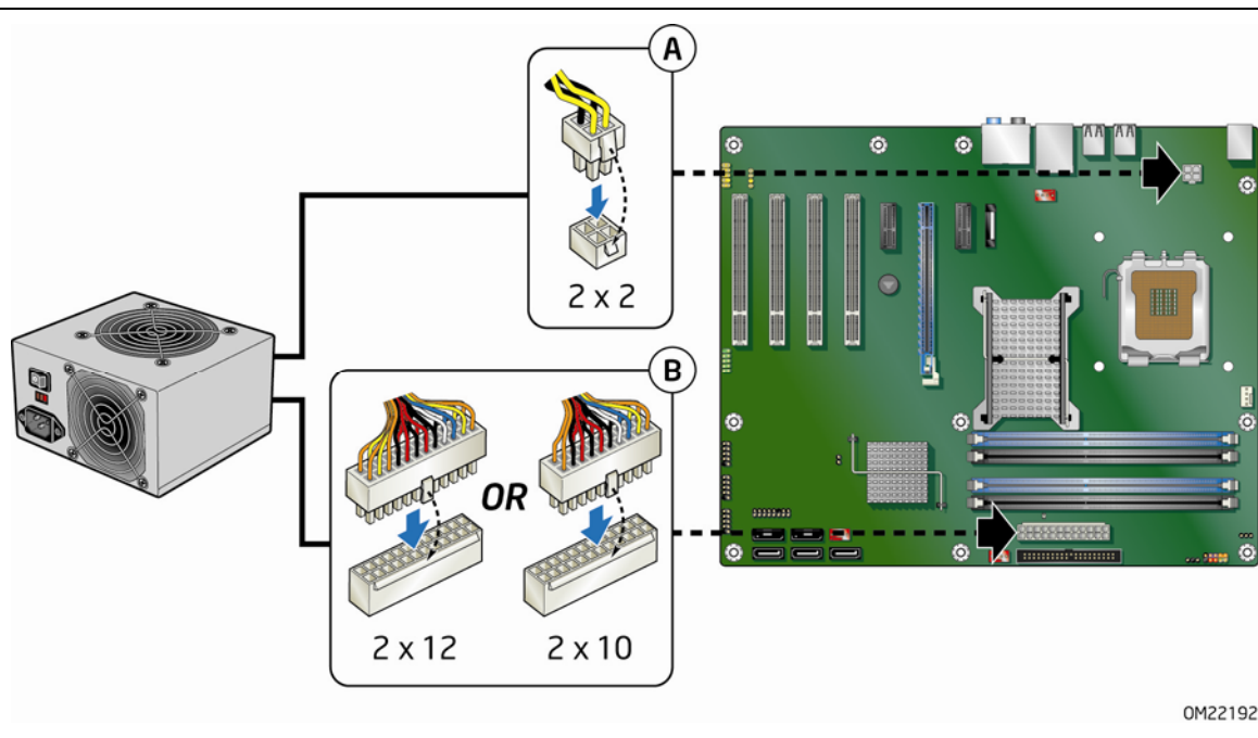
图 25. 连接电源系统电缆
