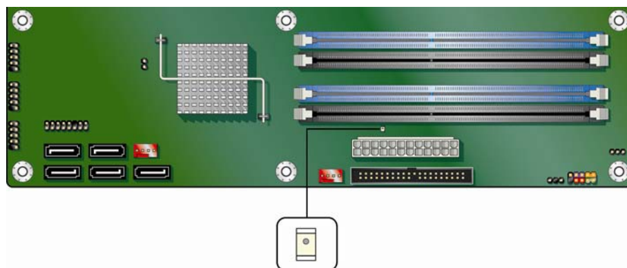
图 3. +5 V 备用电源指示灯位置
