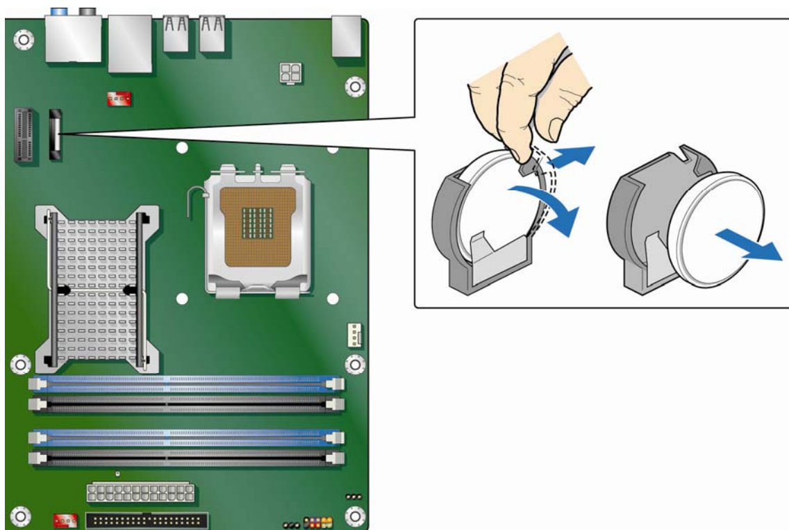
图 27. 拆卸电池
