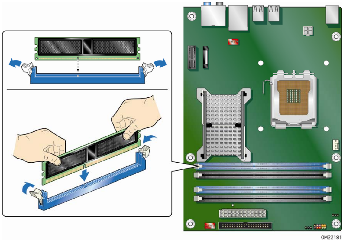
图 17. 安装 DIMM
