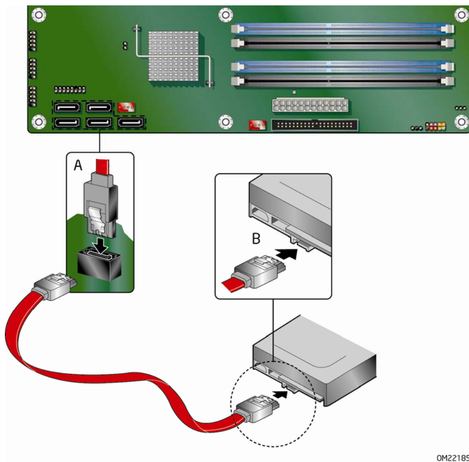
图 21. 连接串行 ATA 电缆
