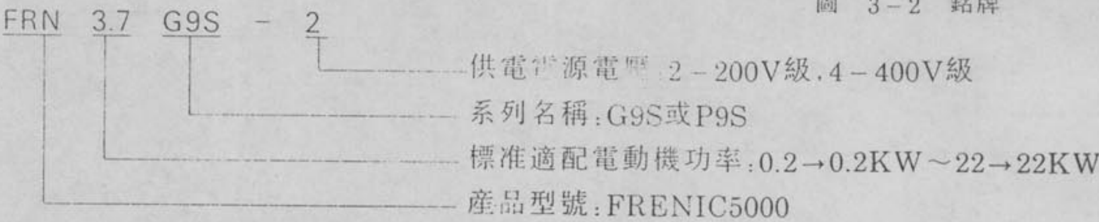
圖 3-2 銘牌
