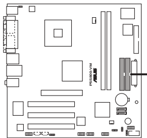
P5S800-VM IDE connectors
