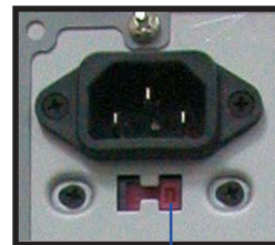
115V/ 230V 電壓選擇開關
