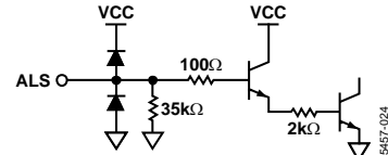
Figure 29. Equivalent Circuit of the ALS Pin
