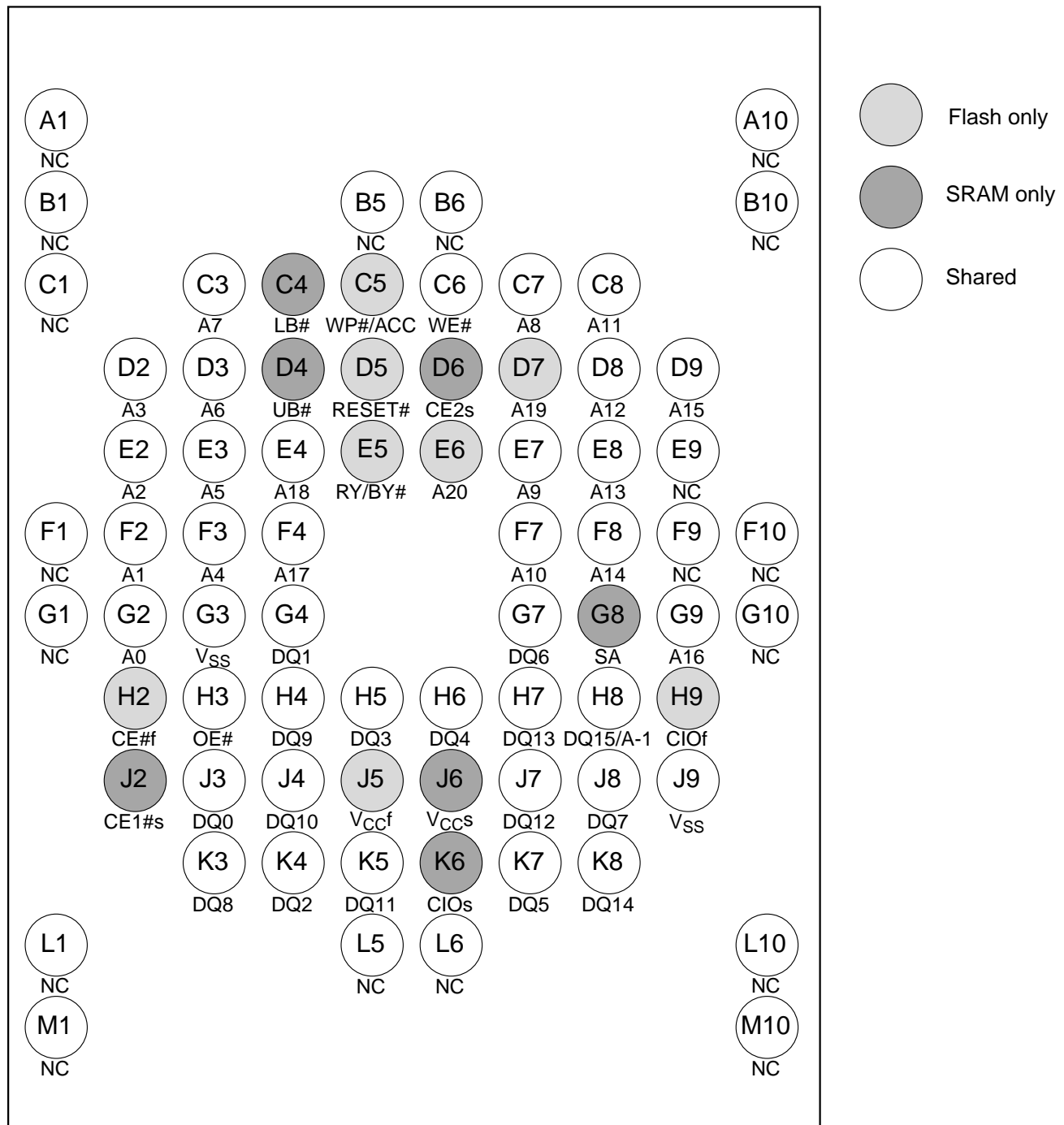
73-Ball FBGA
