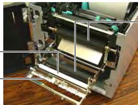
底纸传送轴
