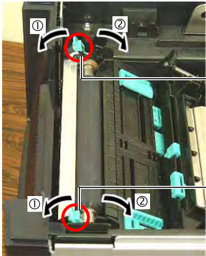
打印头压力调整杠杆
