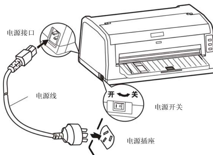
图 2-14 连接电源线
