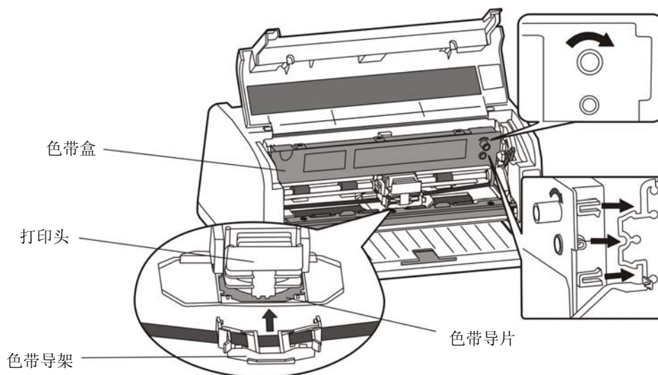
图 2-9 安装色带盒
