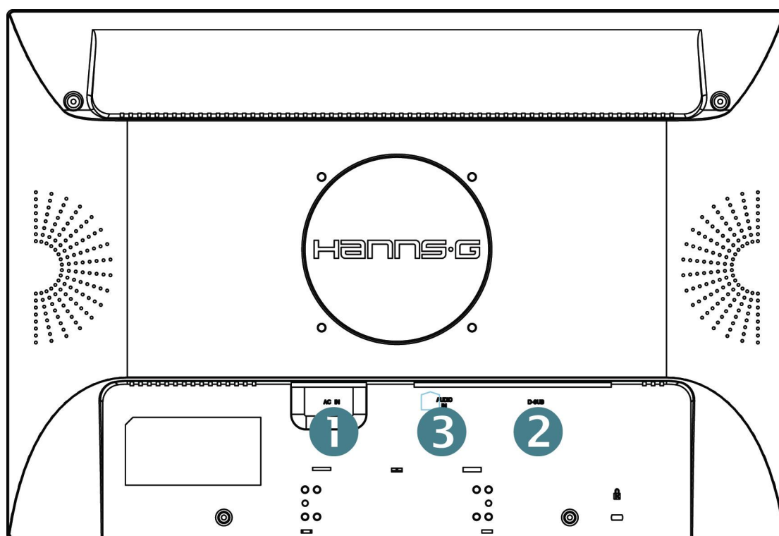
图二. 连接到 PC
