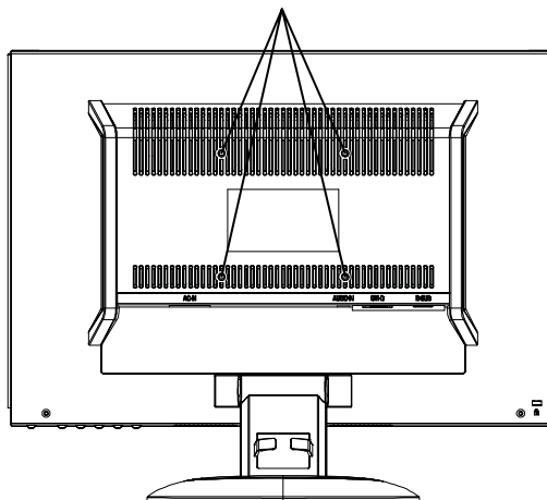
螺絲孔（100 mm x 100 mm）
