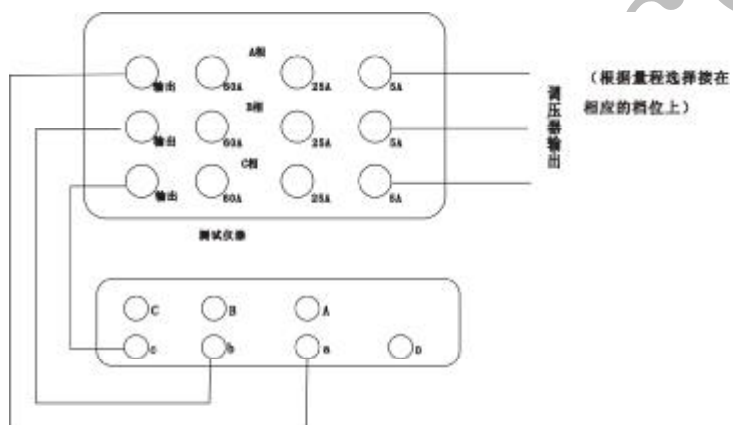
三相变压器空载试验
