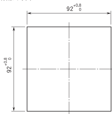
■ 面板切割尺寸图
