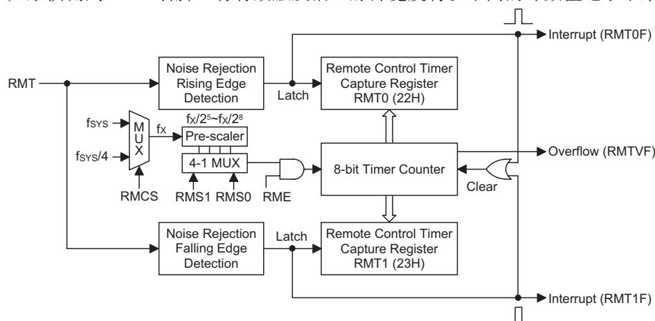
遥控定时器
