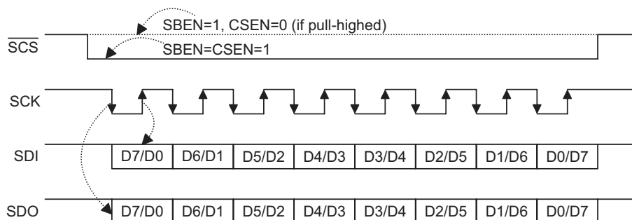
SIO 时序图
