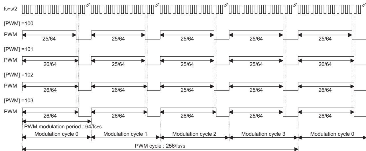
(6+2)位模式 PWM
