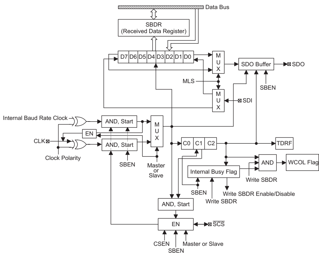
SIO 结构图
