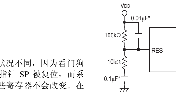
复位电路
