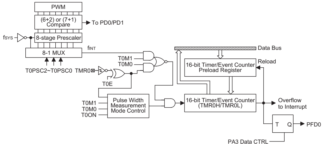
定时/计数器 0
