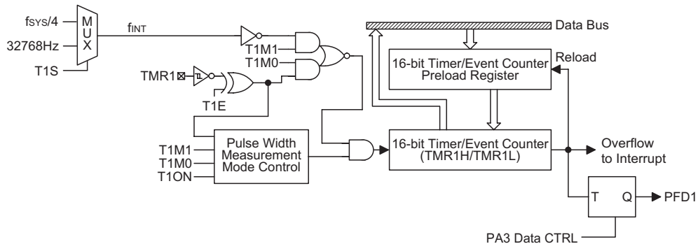
定时/计数器 1
