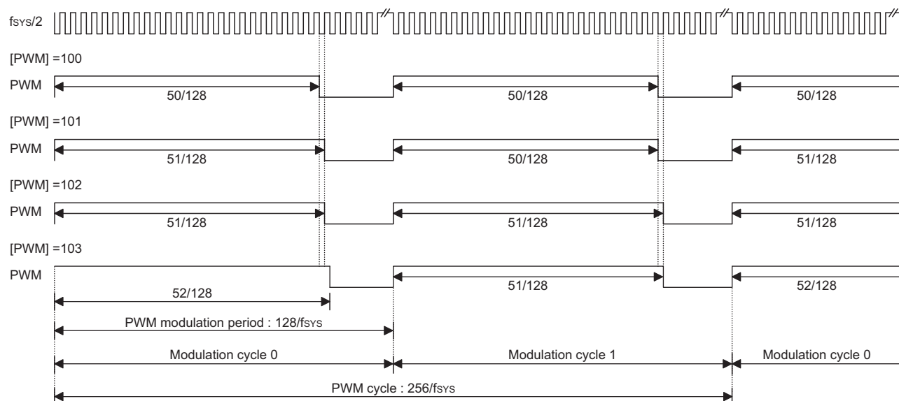
(7+1)位模式 PWM
