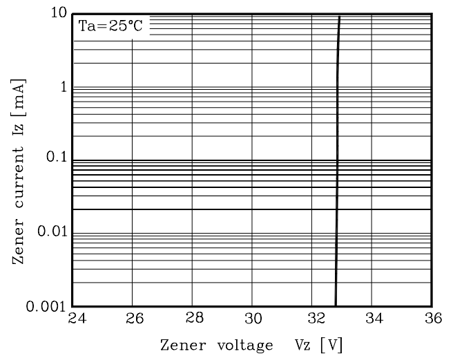
Fig. 2 I_Z - V_Z
