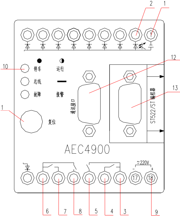
图 1 控制器面板布置图
