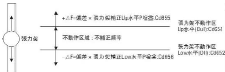
圖 14 張力架補正 3 動作圖
