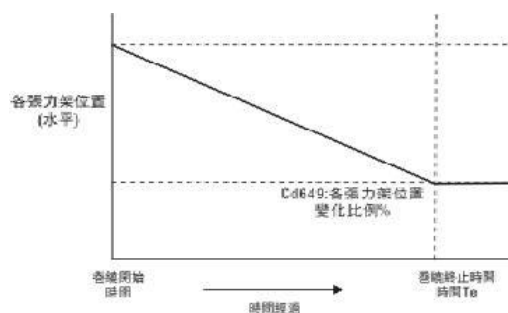
圖 1 2 張力架各位置的变化
