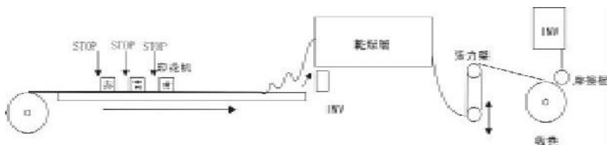
圖 3 印花機卷繞功能系統示例
