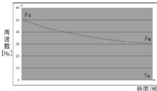
圖2 卷繞曲線例 -
