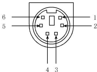
密码键盘接口
