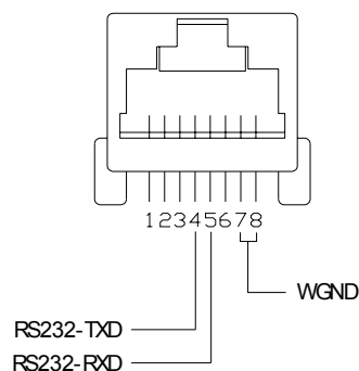
图 2-2 RS-232 信号定义
