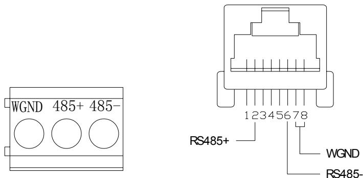
图 2-3 RS-485 两种连接方式信号定义
