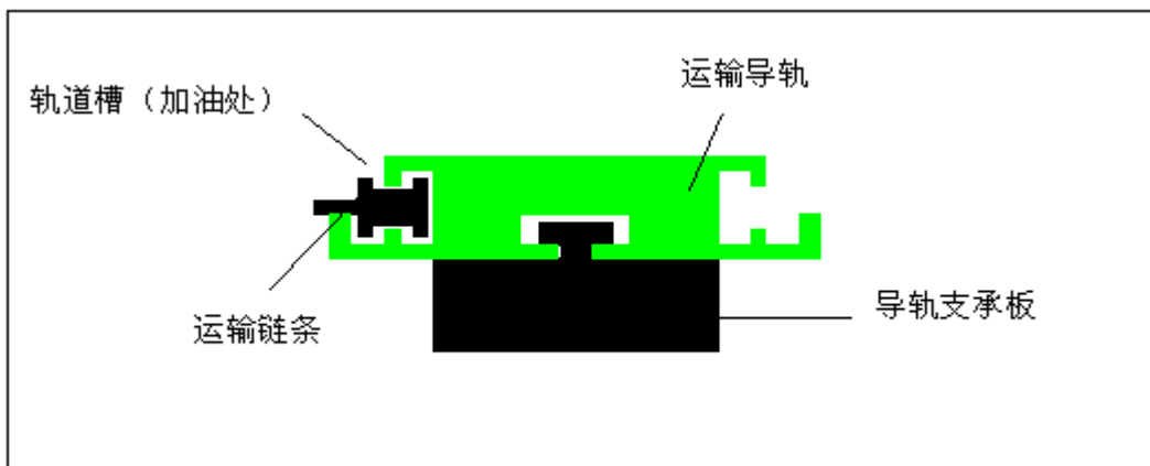
图 7-1 清洁运输链条
