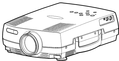
LCD Projector with lens cap LCD Projektor mit Schutzkappe Projecteur LCD avec protection lentille Projector LCD con tapa del lente Proiettore LCD con coperchietto Projektor LCD con protetor de lente LCD-projektor med linsedeksel
