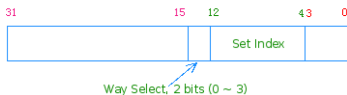
Figure 8: Indexed 方式地址分解
