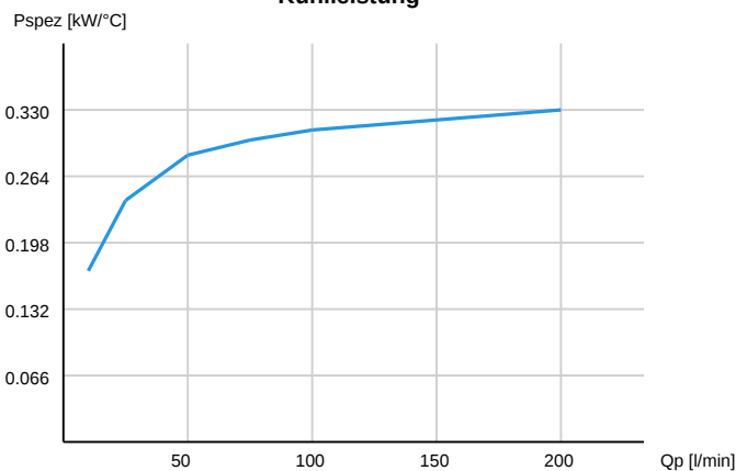
Kühlleistung*
