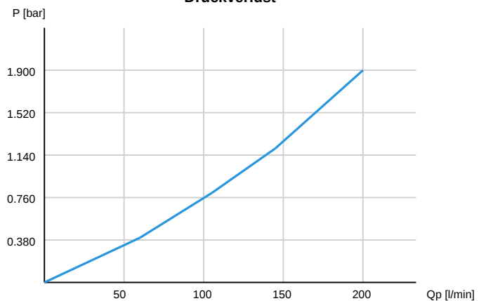
Druckverlust
