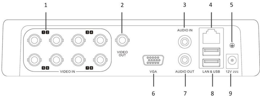
接口示意图
