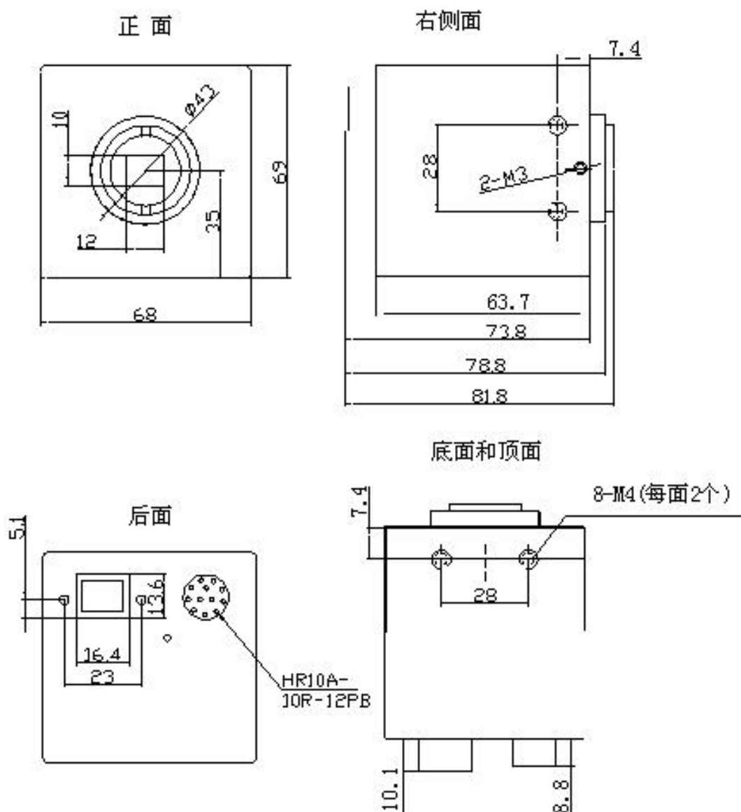
图 2 MVC610DAM-GE110 的外形尺寸图
