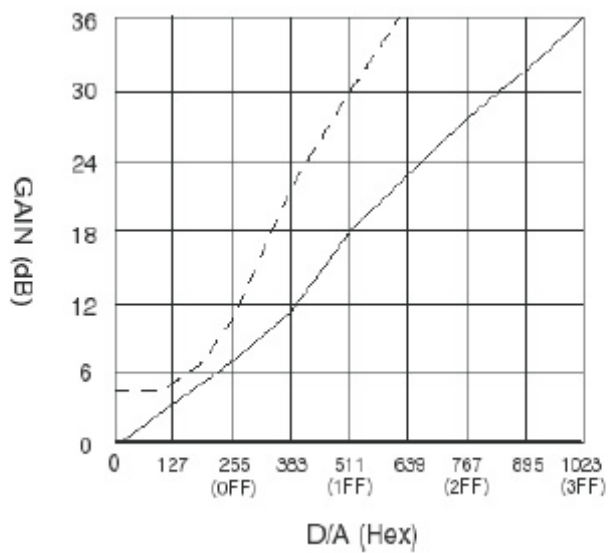
图 4 MVC610DAM-GE110 增益控制曲线
