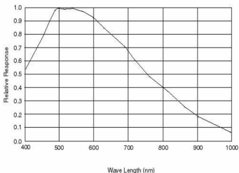
图 1 MV610DAM-GE110 的光谱曲线
