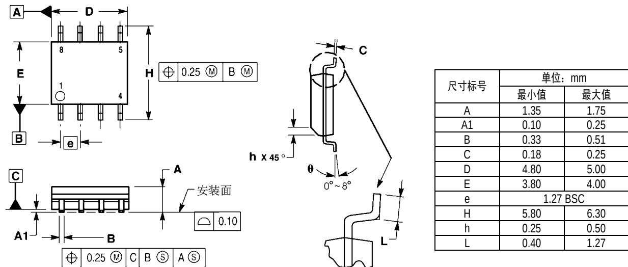
图 7 SOP8 封装外形尺寸图
