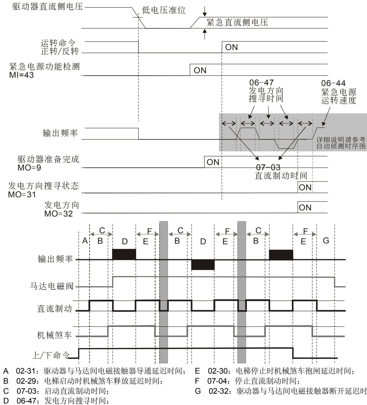
自动侦测时序图
