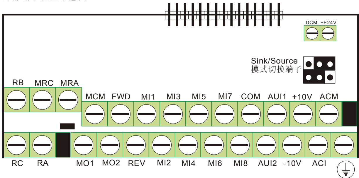
外部端子位置示意图
