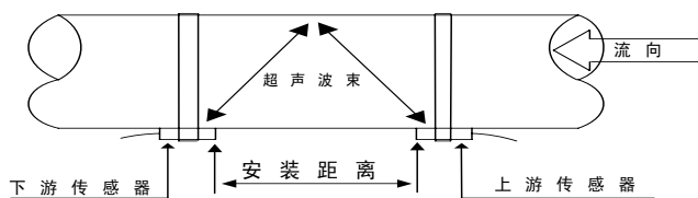
V 法——截面图
