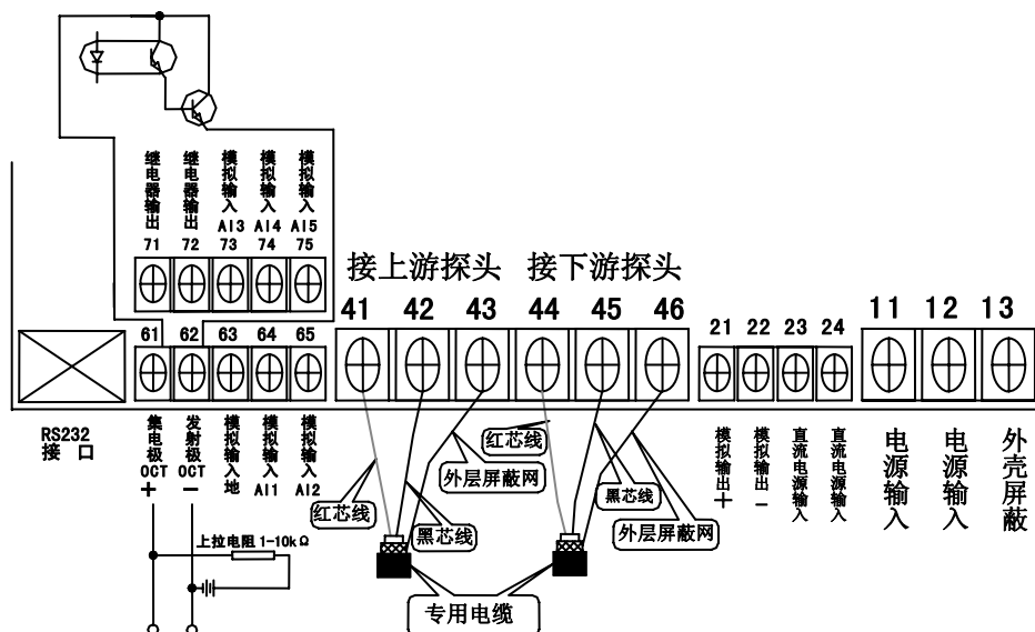
固定式标准型（AFVF1）主板接线图
