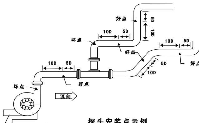
探头安装点示例
