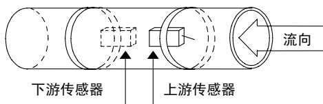
Z 法 —— 侧视图
