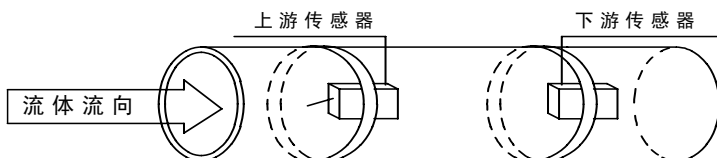
W 法 —— 侧视图
