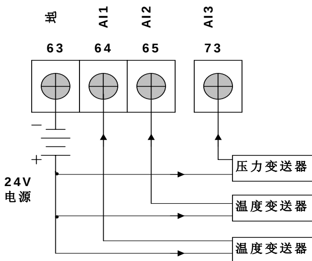
模拟输入接线示意图
