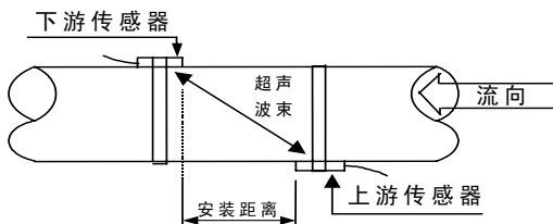
Z 法 —— 顶视图
