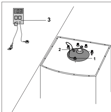
图 6.1 镁保护阳极棒的维护
