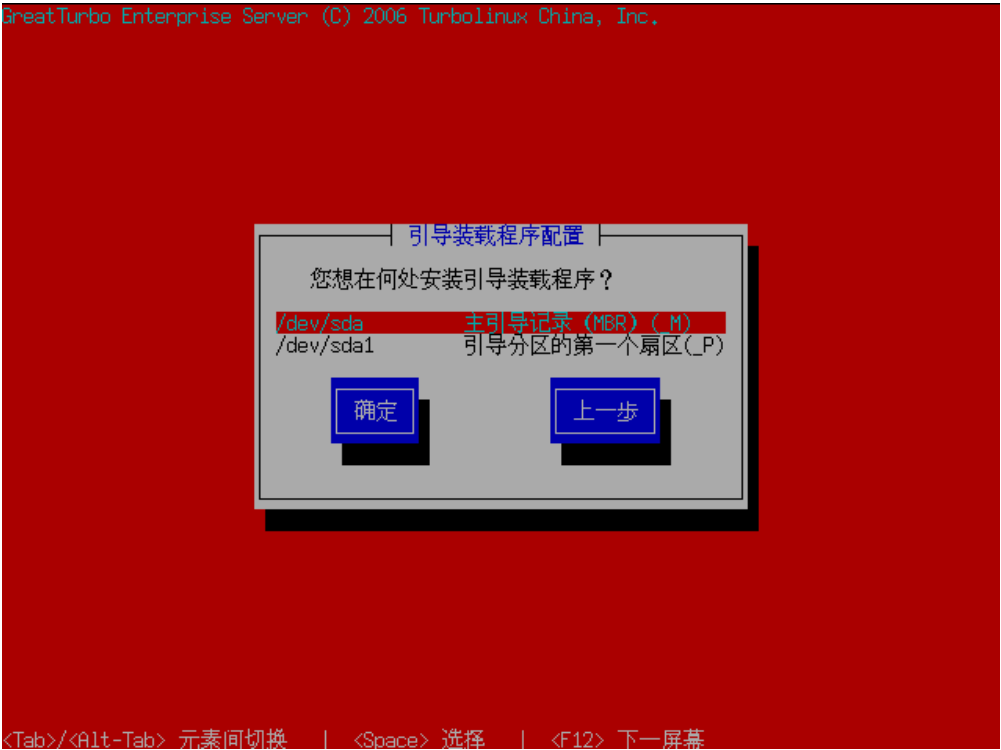
图 B-15 引导装载程序配置—在何处安装引导程序
