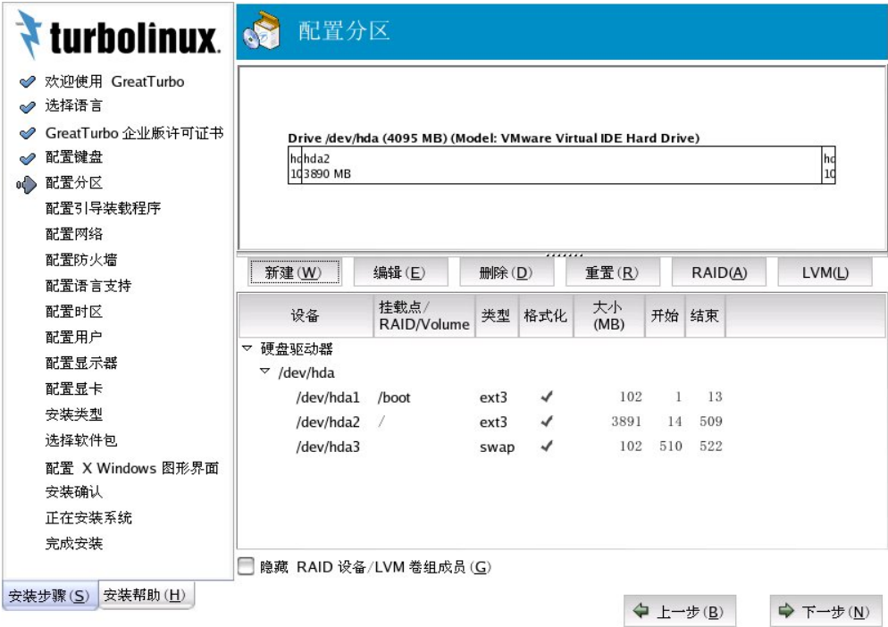
图 3-12 使用 Disk Druid 配置分区后的情况
