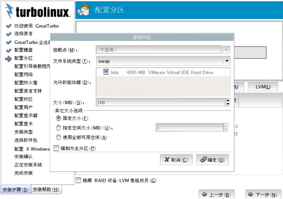
图 3-11 使用 Disk Druid 添加 swap 分区
