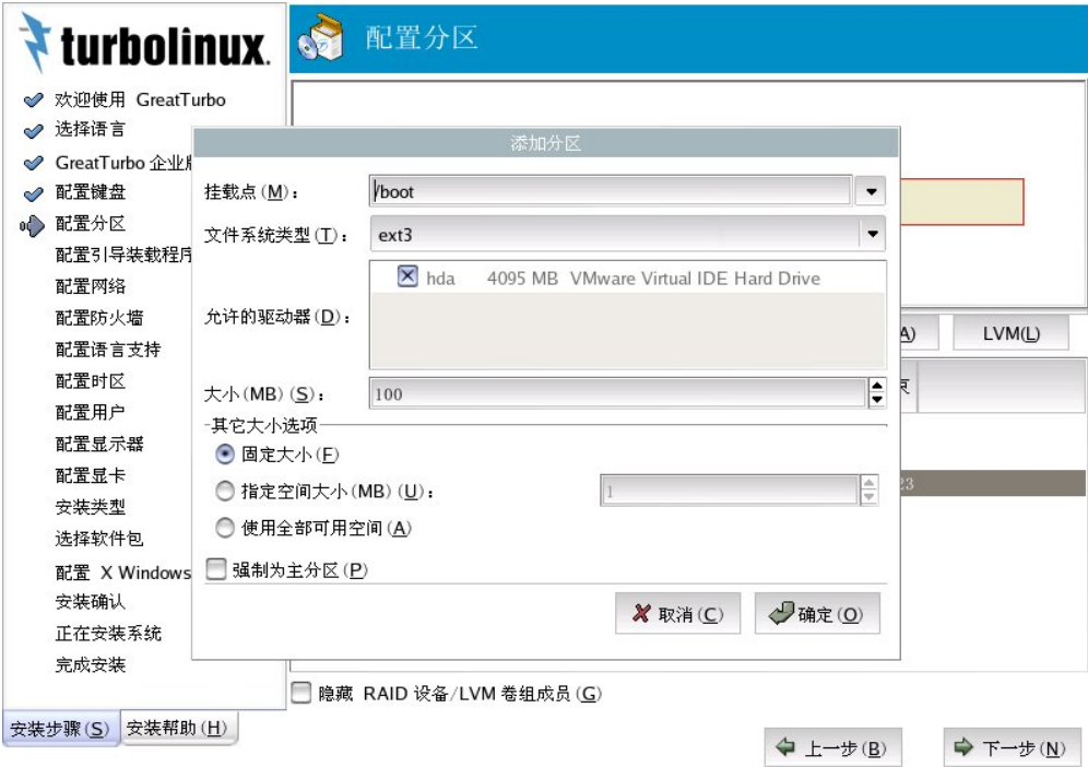
图 3-9 使用 Disk Druid 添加/boot 分区
