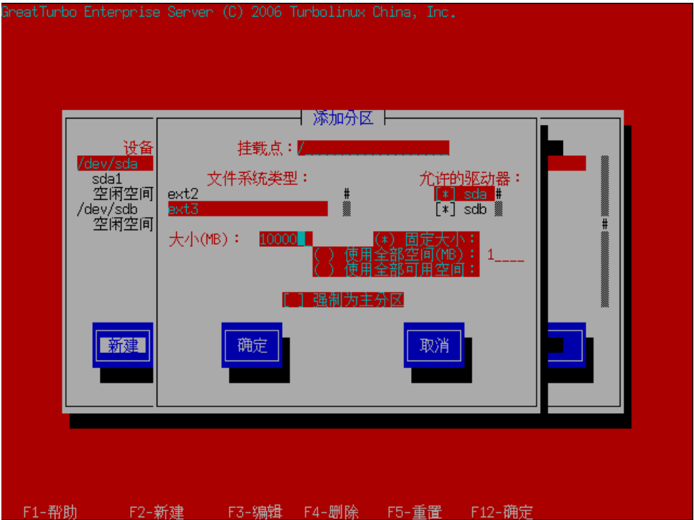
图 B-10 手动分区方式一添加 / 分区
