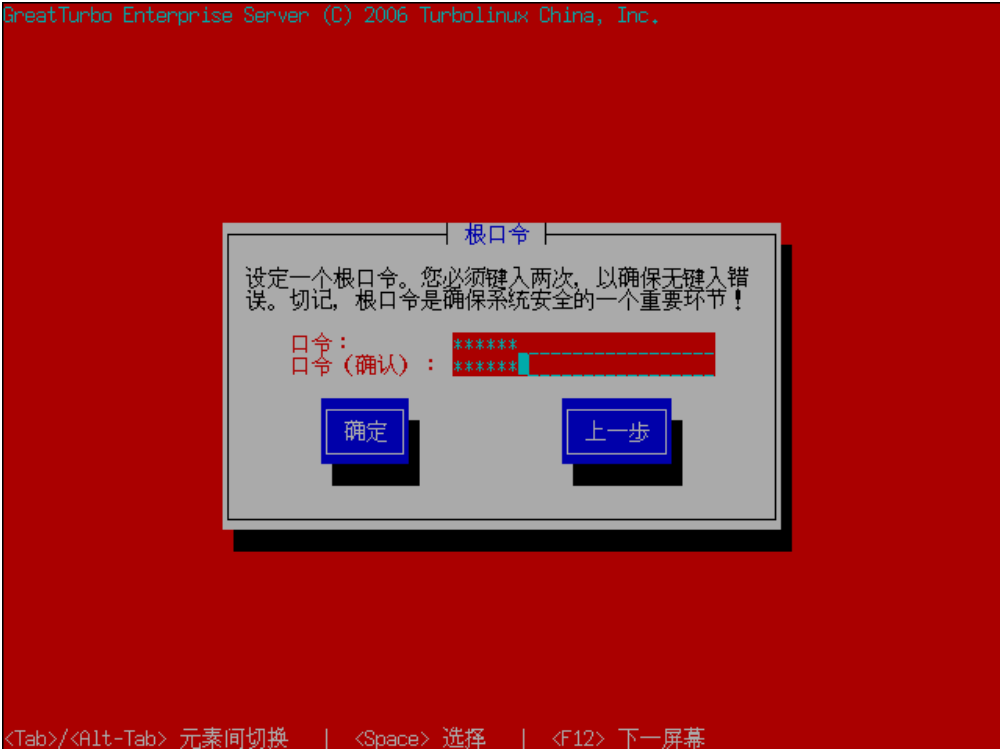
图 B-23 设置根口令
