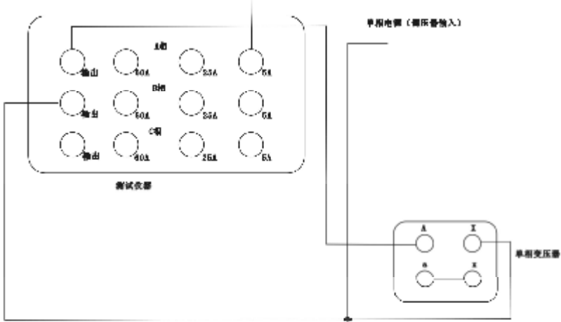
单相变压器负载试验
