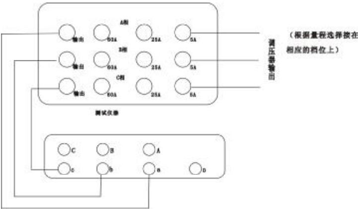
三相变压器空载试验
