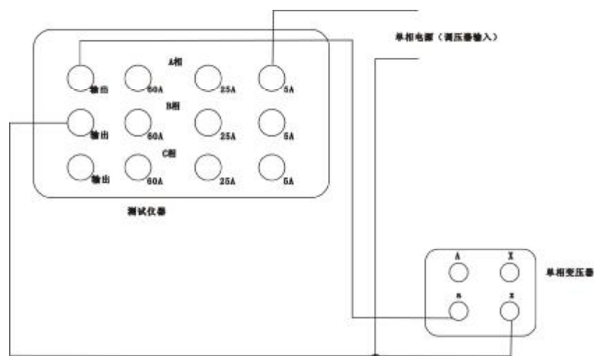
单相变压器空载试验
