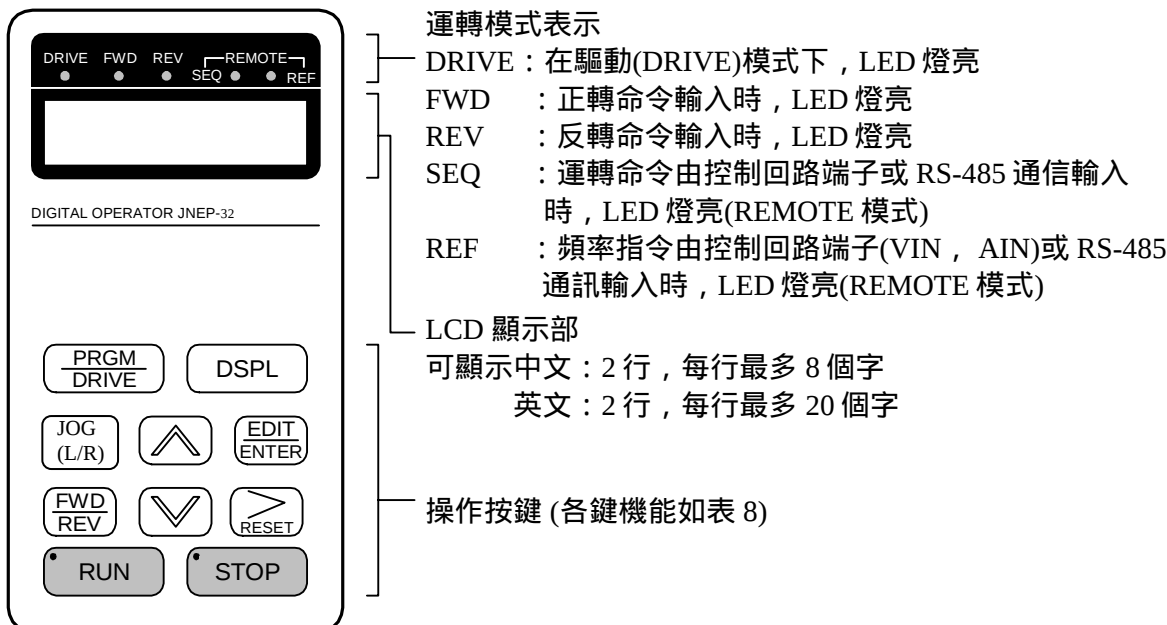
圖 9-a LCD 操作器各部名稱及機能
