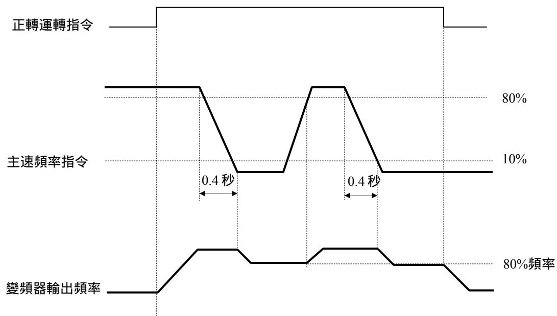
時序圖
