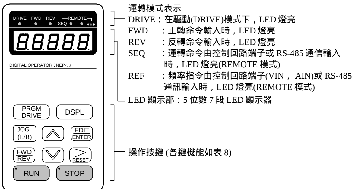
圖 9-b LED 操作器各部名稱及機能
