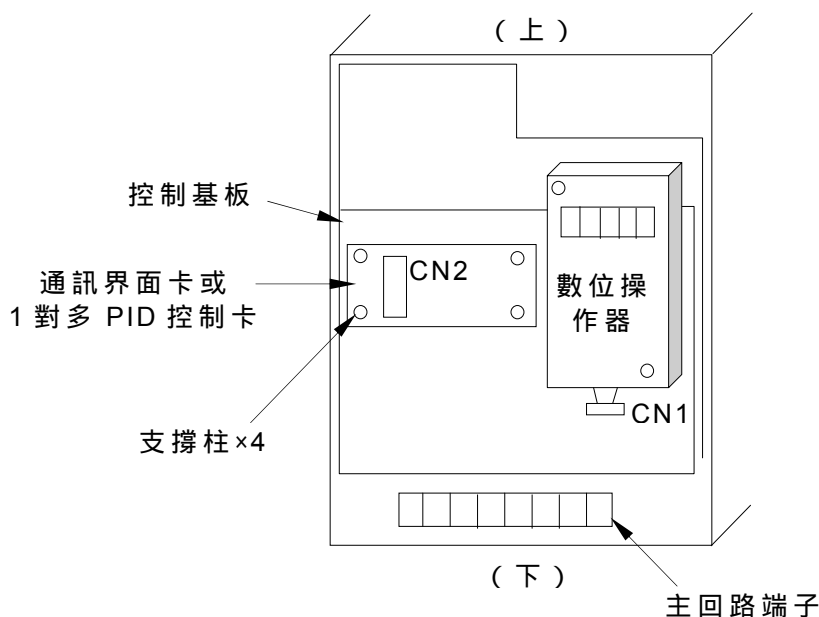
圖 8 界面卡安裝方式
