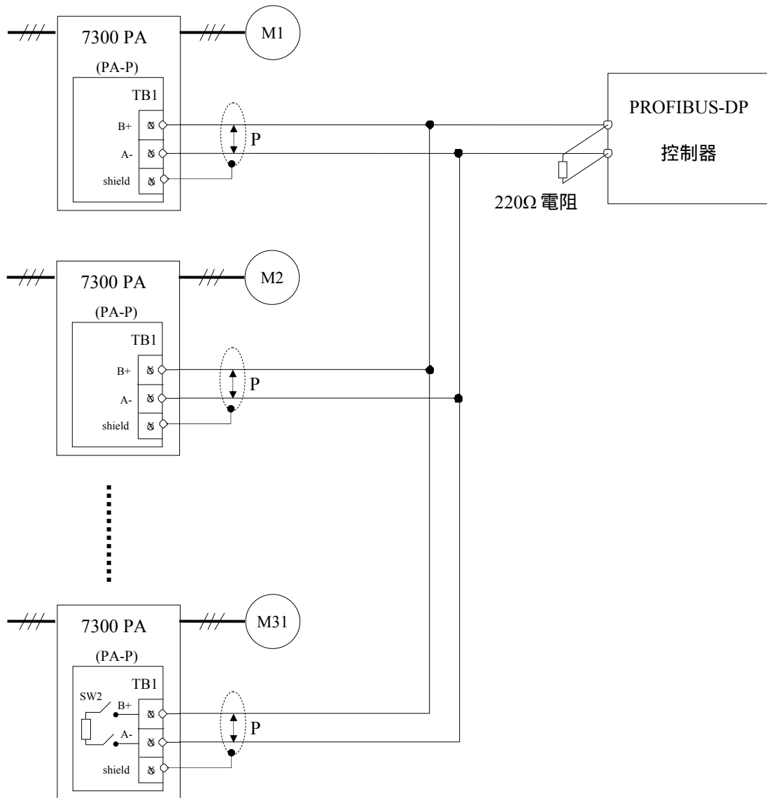
圖 17 PROFIBUS 通訊界面卡配線
