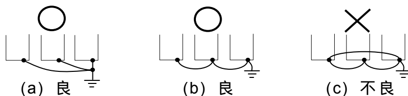
圖 4 7300PA 多台接地方法
