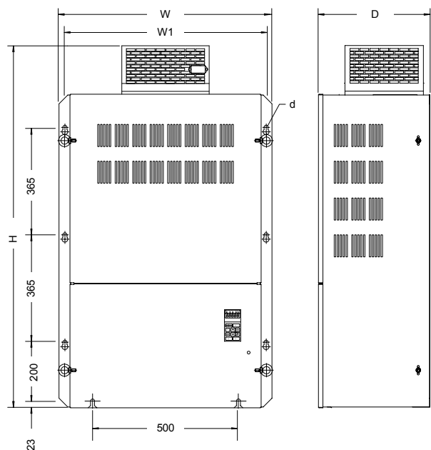
( 盤內安裝型 - IP00 )
