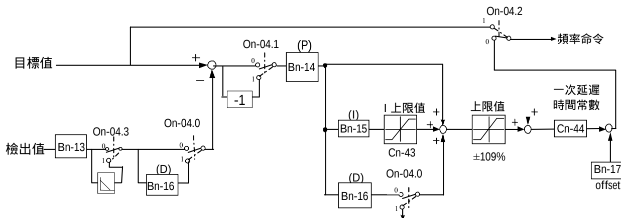
圖 11-(b) PID 控制方塊圖 (Ver : 04xx 以後)
