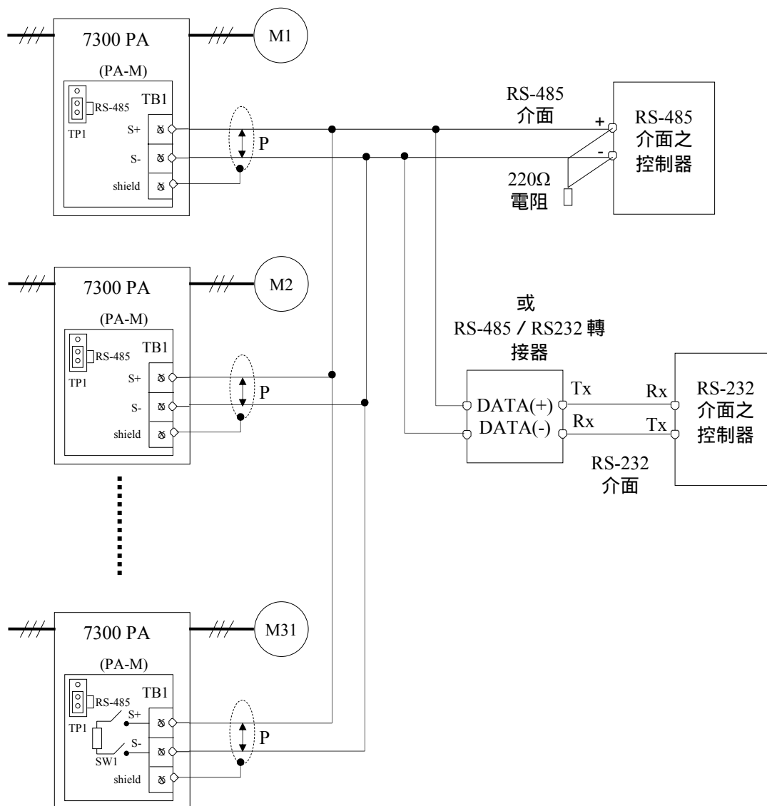
圖 16 MODBUS 通信界面卡配線
