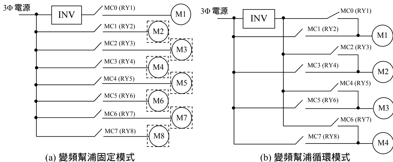
圖 14 變頻幫浦驅動模式
