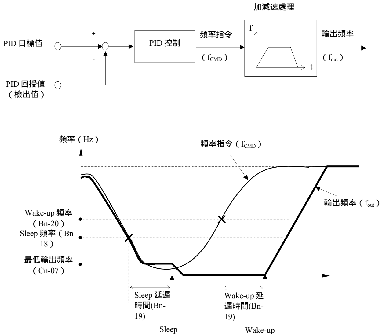
圖 12 PID Sleep / Wake-up 動作
