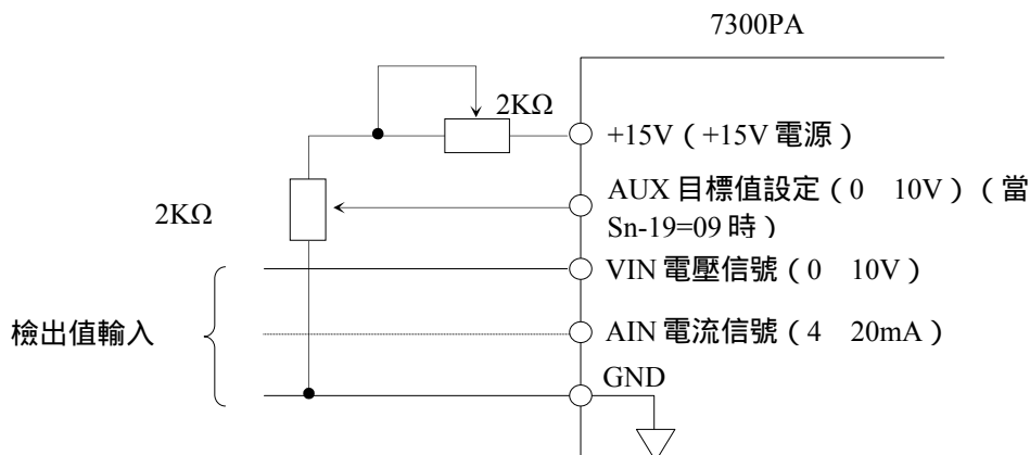
圖 15 PID 控制信號輸入
