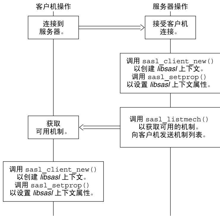
图 7-3 SASL 会话初始化
