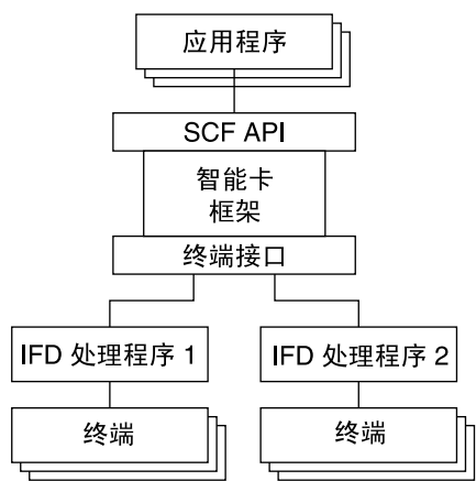
图 10-1 智能卡框架
