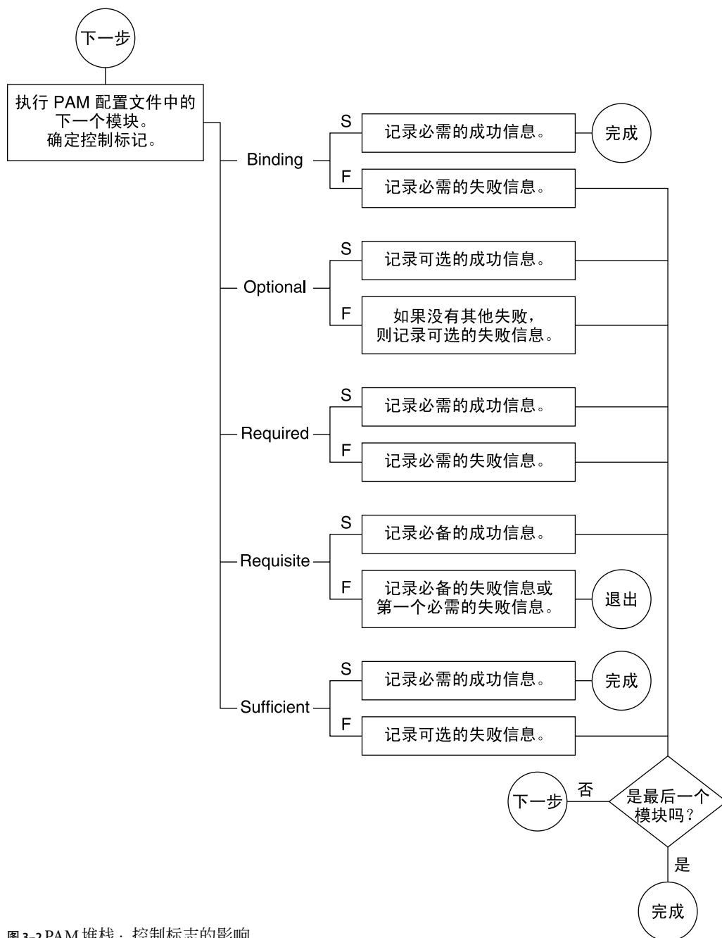
图 3-2 PAM 堆栈：控制标志的影响
